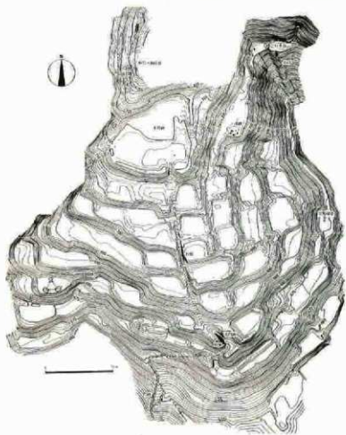
第12図 弥高寺跡測量図
