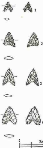
第22図 伊吹山頂遺跡出土石器実測図
