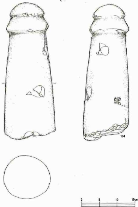
第47图 杉沢遺跡出土石器実測图 ⑤
