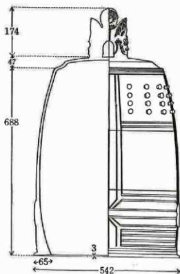
第23図 松尾寺遺跡出土梵鐘実測図(文献19)
