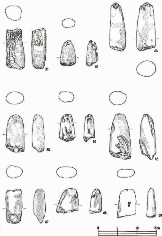
第44圖 杉沢遺跡出土石器実測圖 ㊸
