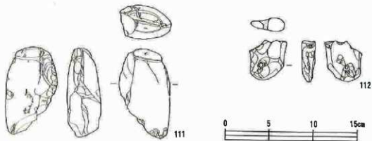
第48圖 杉沢遺跡出土石器実測圖
