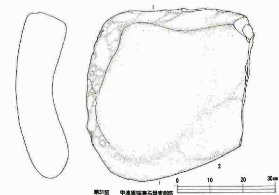
第31图 甲津原採集石器実測图
