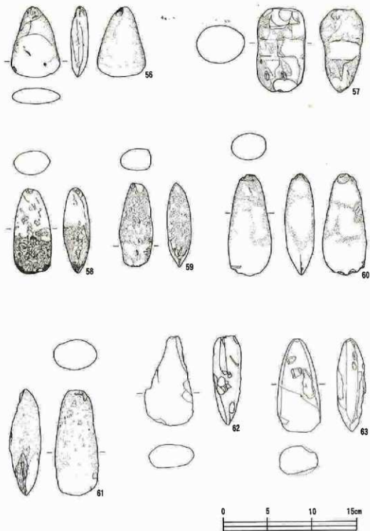
第41图 杉沢遺跡出土石器実測图 ㊸
