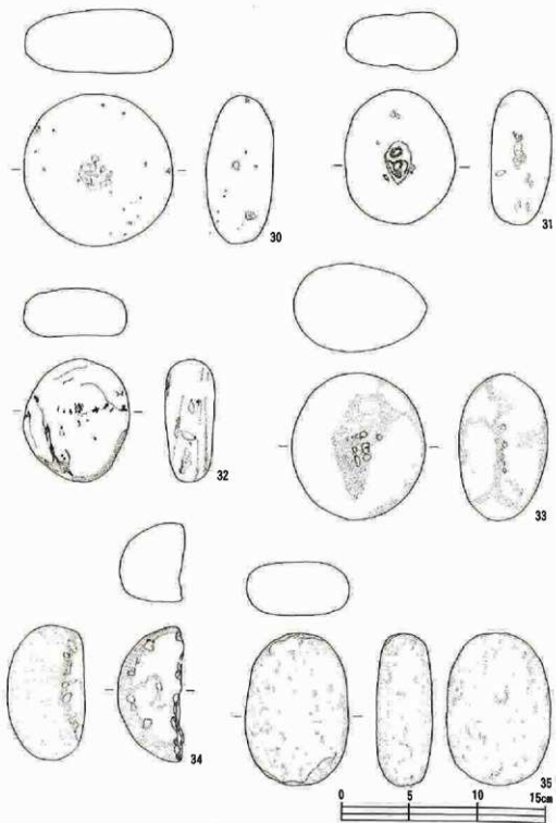
第38図 杉沢遺跡出土石器実測図 ⑥
