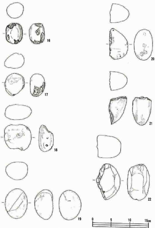
第36圖 杉沢遺跡出土石器実測図 ④
