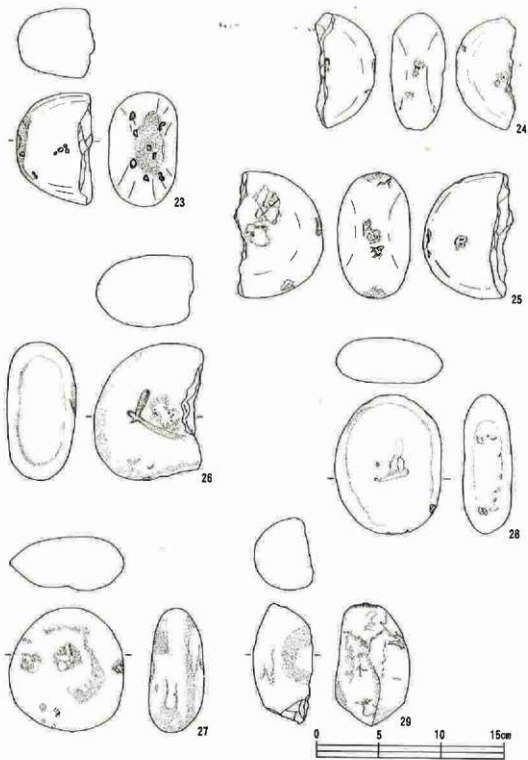
第37図 杉沢遺跡出土石器実測図 ⑤
