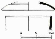
第24図 赤谷遺跡出土土器夾測図
