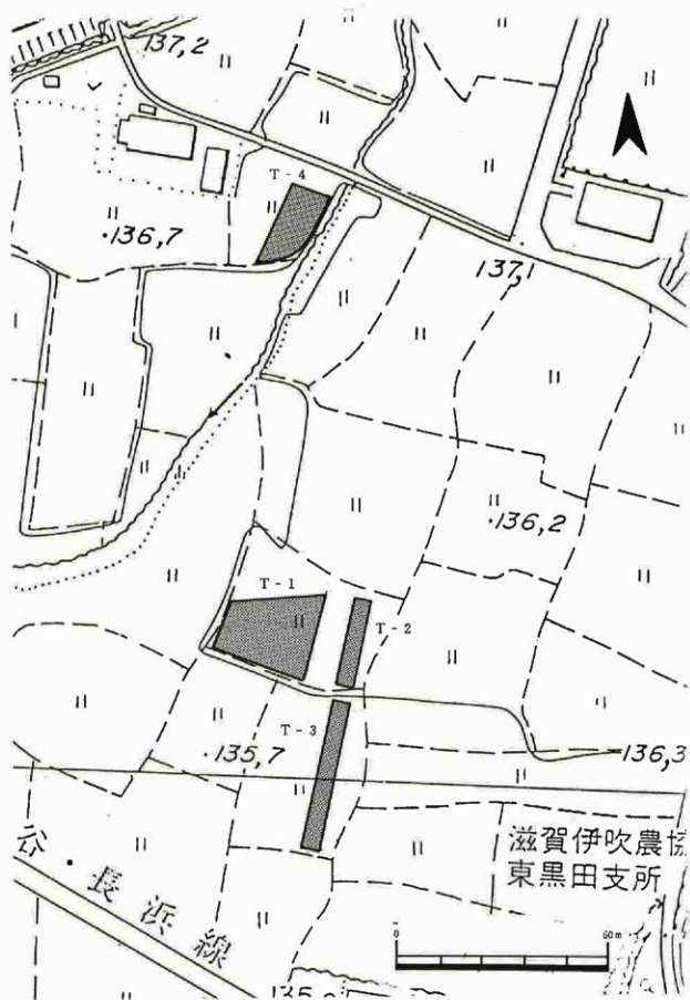
図2 ドレン配置図
