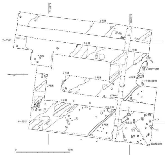
第4図 遺構配置図 (1/200)
