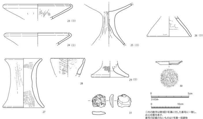
第11図 1号溝出土遺物実測図② (1/4・2/3)
