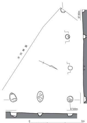
第8図 掘立柱建物実測図（1/60）
