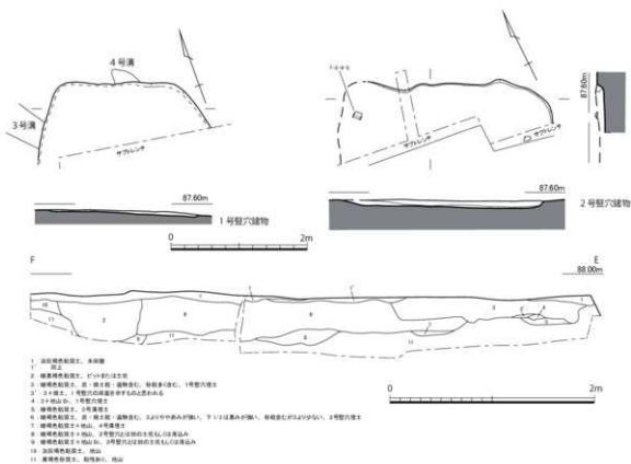
第6図 1・2号型穴建物および型穴建物周辺土層実測図 (1/60、土層は1/40)
