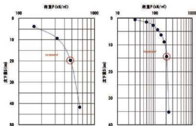
図3-18 平板載荷沈下量関係曲線(左1号墳:右2号墳)
