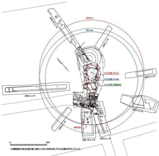
図 3-27 1号墳全体調査区配置図 (1/250)
