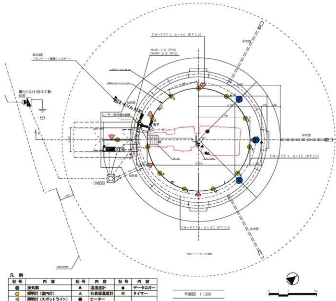
図4-7 電気設備等平面図 (1/200)
