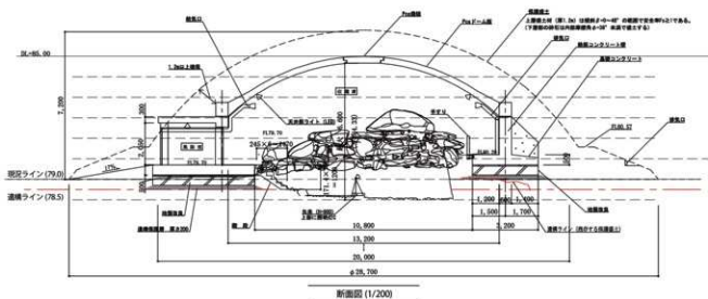
図 4-2 断面図
