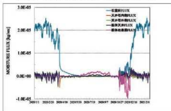
図 3-12 各境界の水分フラックス（地表断湿）
