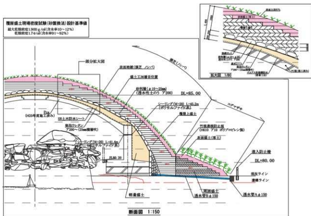
図 4-10 盛土施工断面図 (1/80・150)
