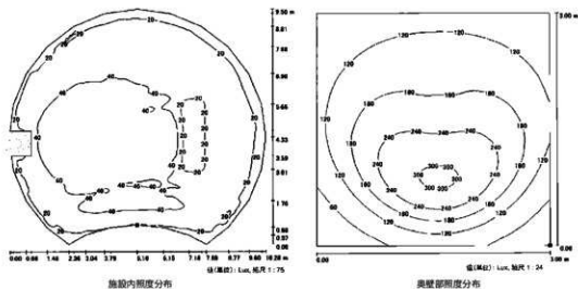
図 4-8 照度分布計画図
