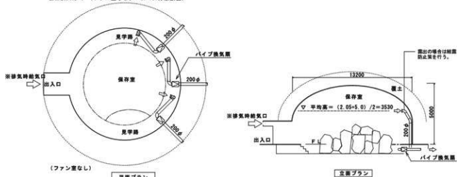
図 4-9 換気設備計画模式図
