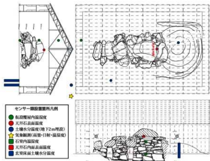
図3-1 環境調査箇所位置図 (1/250)
