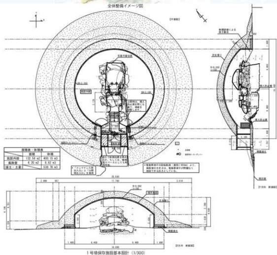
図2-4 整備基本計画イメージ図
