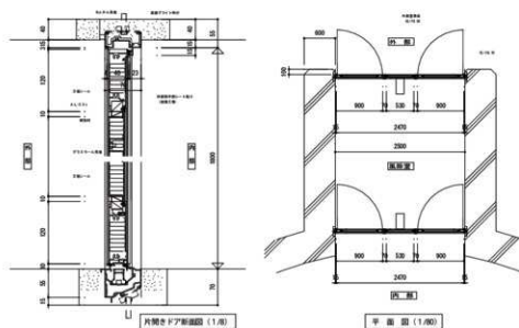
図4-6 建具平面図 (1/8・1/80)
