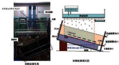
図3-21 キャピラリーバリア実験装置
