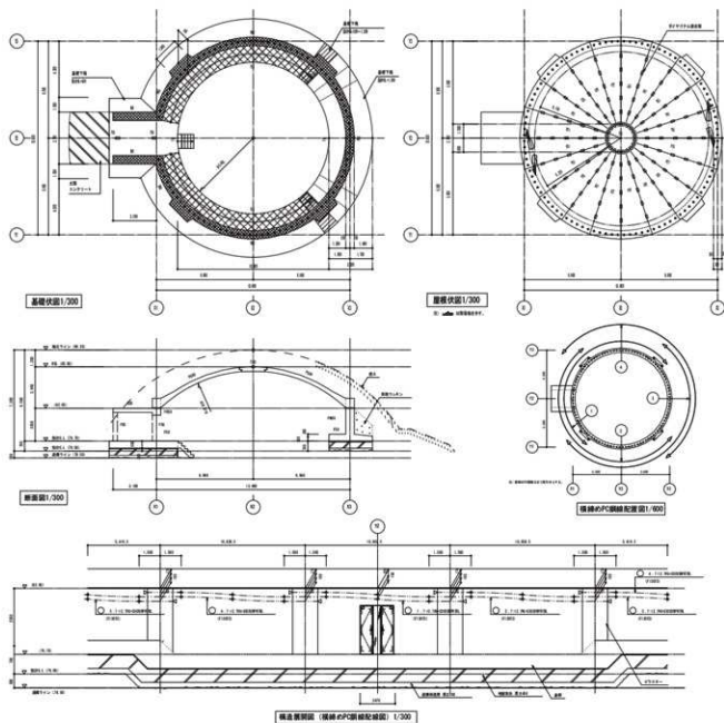
図4-5 構造図 (1/300・1/600)
