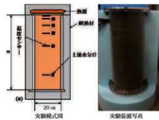
図3-22 熱遮断実験装置
