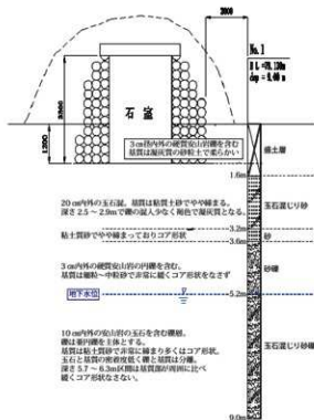
図 3-17 地質断面図
