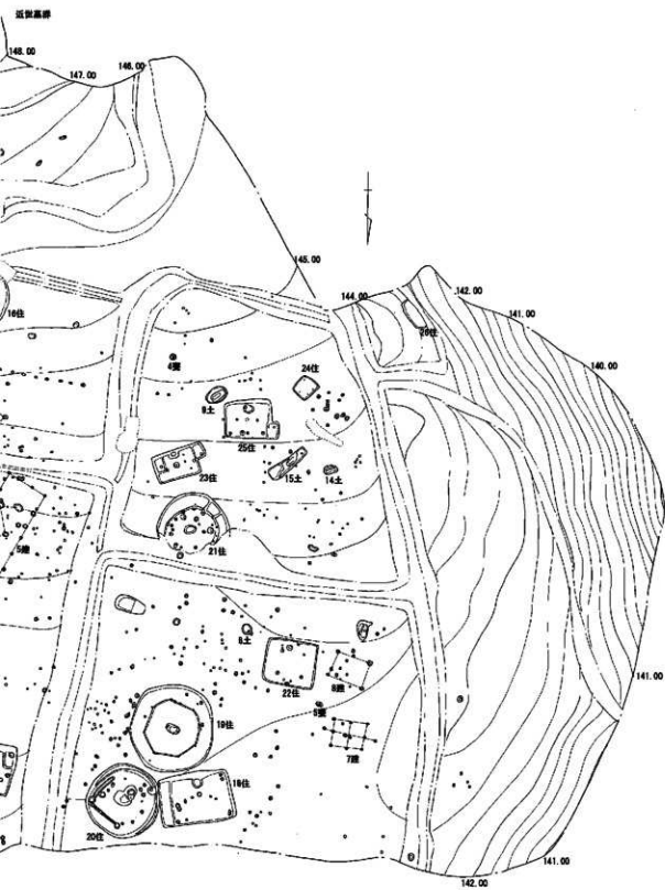
配置圖 (1/500)
