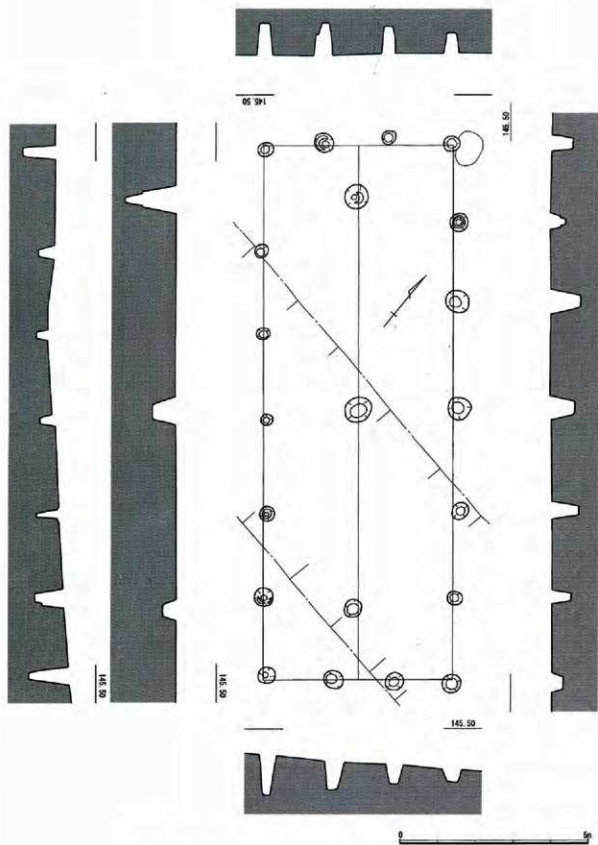
第 31 图 4 号掘立柱建筑物实测图 (1/100)
