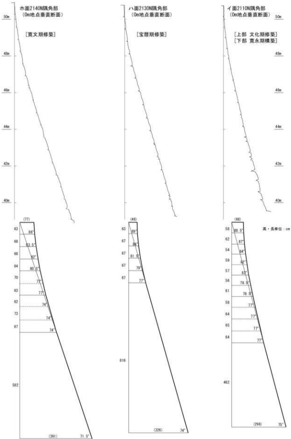
第220図 石垣勾配の比較 (S=1/100)
