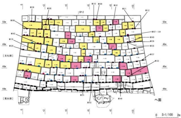
第214図 押石・敷金等使用色分け図 10 イ (2110N)・ハ面 (2110E) (S=1/100)
