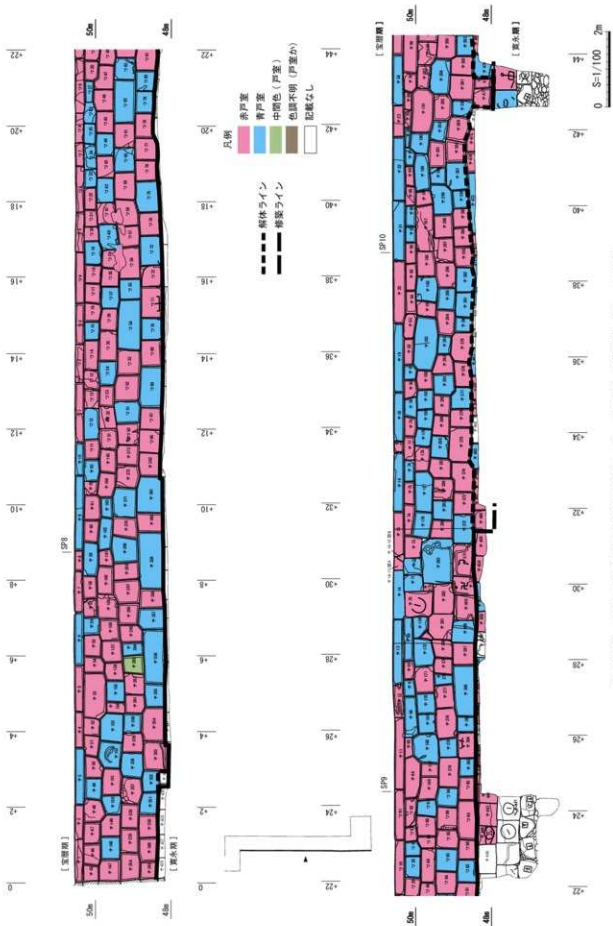
第 197 図 石材（色調）別色分け図 8 チ・ヲ面北（2120W）（S=1/100）
