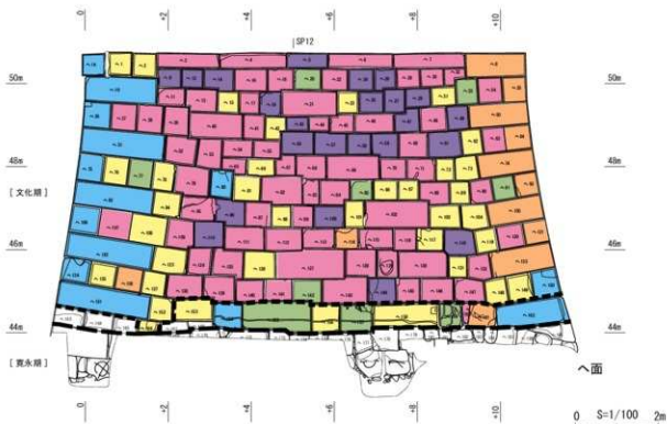
第177図 控え長別色分け図10 イ (2110N)・へ面 (2110E) (S=1/100)
