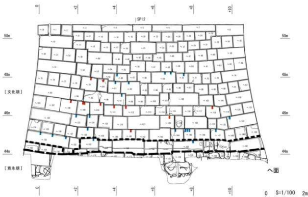
第203図 「榻子穴」立面投影図3 イ (211N)・ハ面 (211E) (S=1/100)
