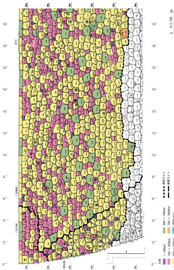
第183図 面面積別色分け図5 ロ面南 (2120E) (S=1/100)
