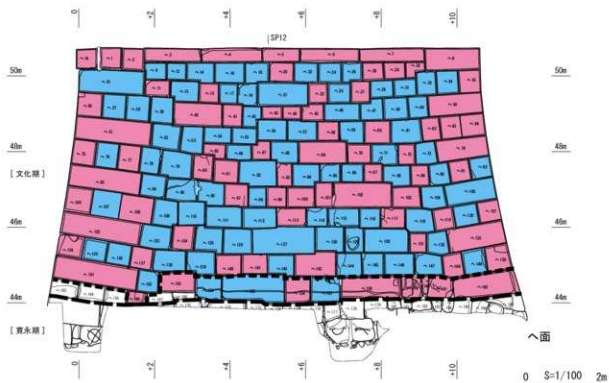
第199図 石材(色調)別色分け図10 イ(2110N)・へ面(2110E)(S=1/100)
