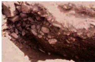
五十間長屋台東西土層断面 SP10北6.5m地点 L=50.4_49.2m付近南壁
