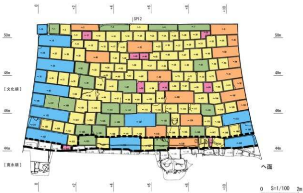
第188図 面面積別色分け図10 イ (2110N)・へ面 (2110E) (S=1/100)
