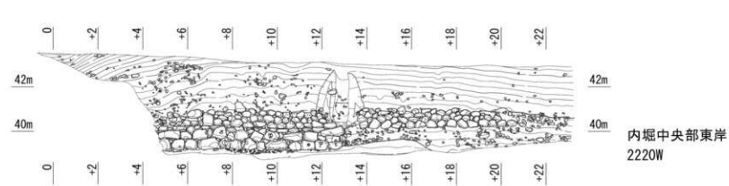
石垣立面图 1 (S = 1/150)
