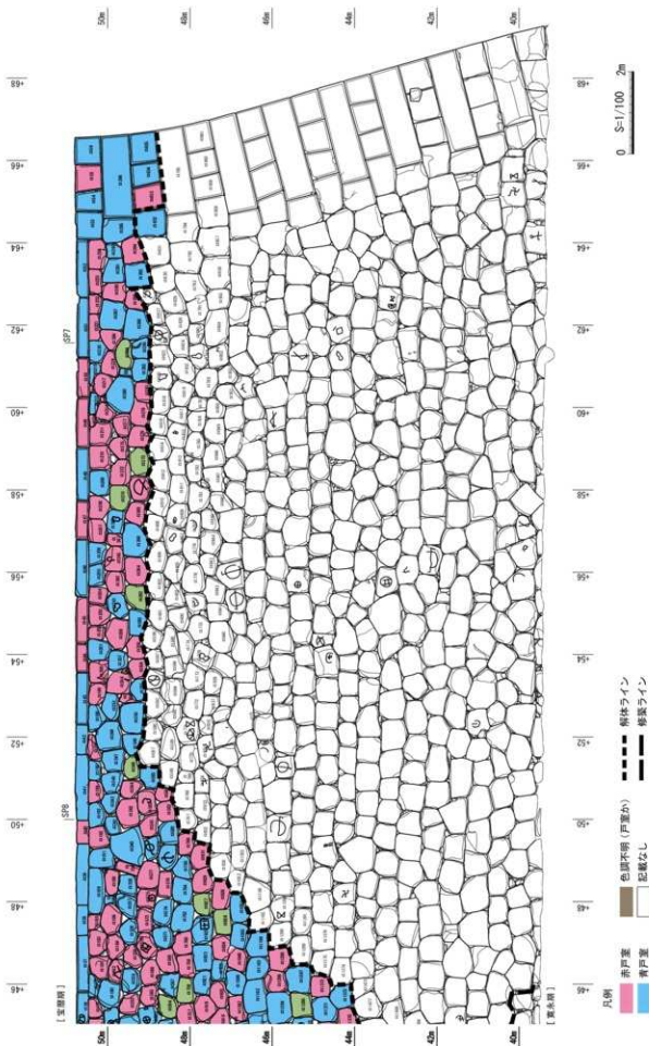
第196図 石材(色調)別色分け図7 口面北(2120E) (S=1/100)
