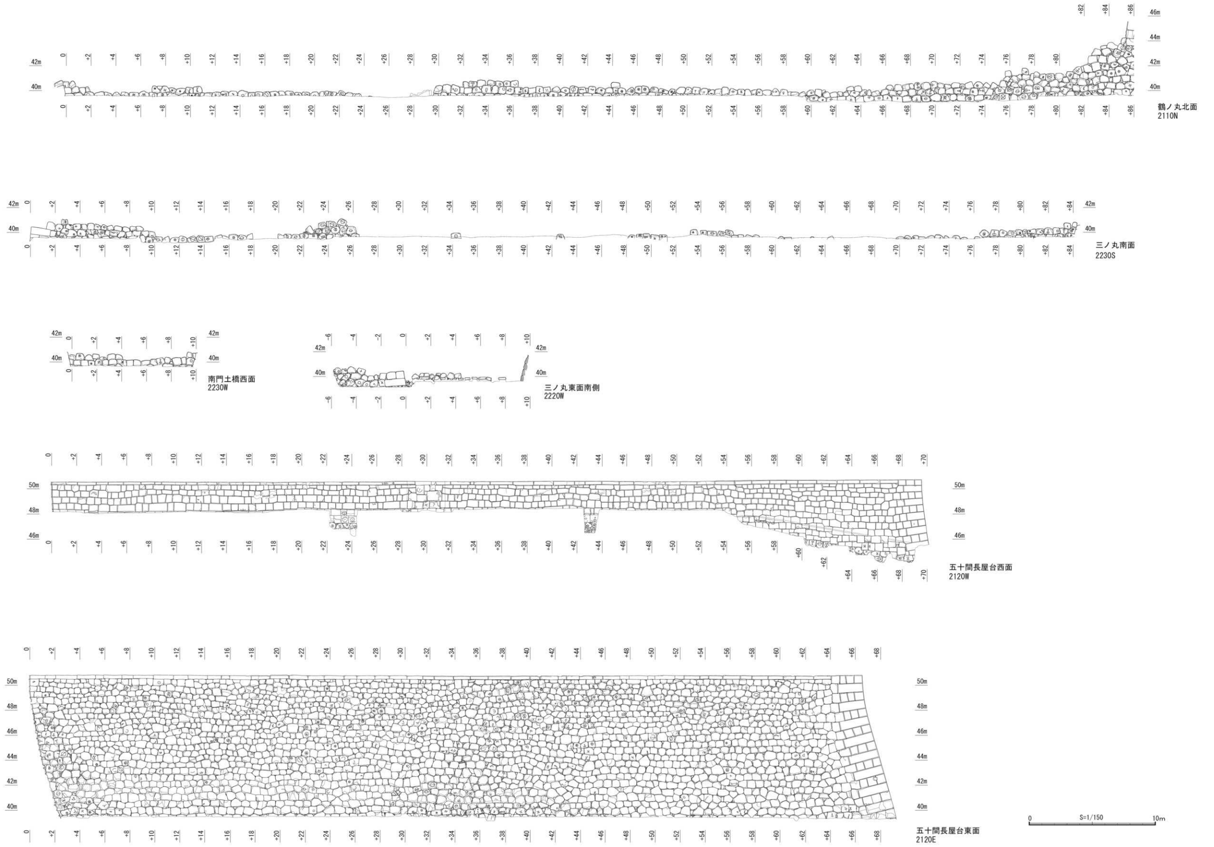
石垣立面图2 (S=1/150)
