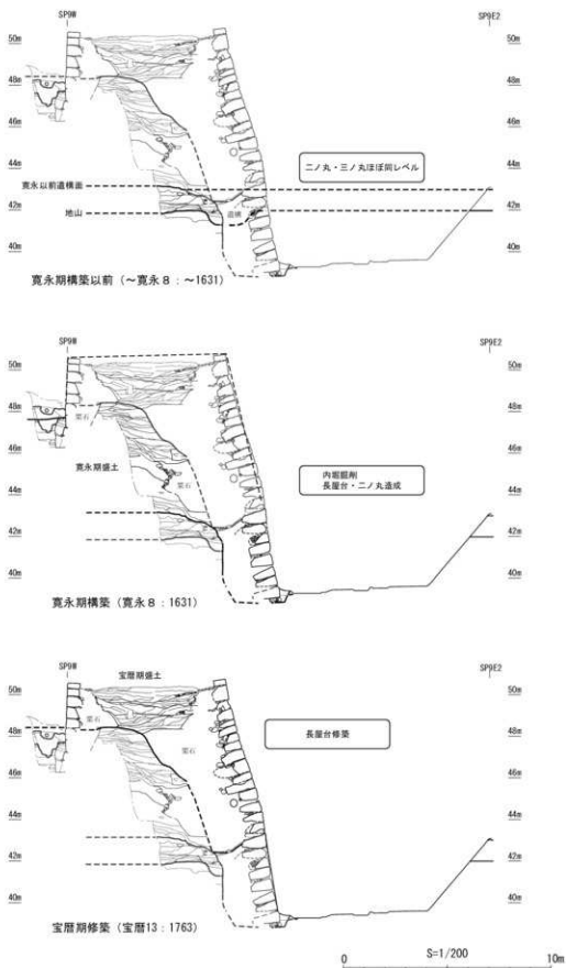
第222図 五十間長屋台・内堀の構築・修築過程 (S=1/200)
