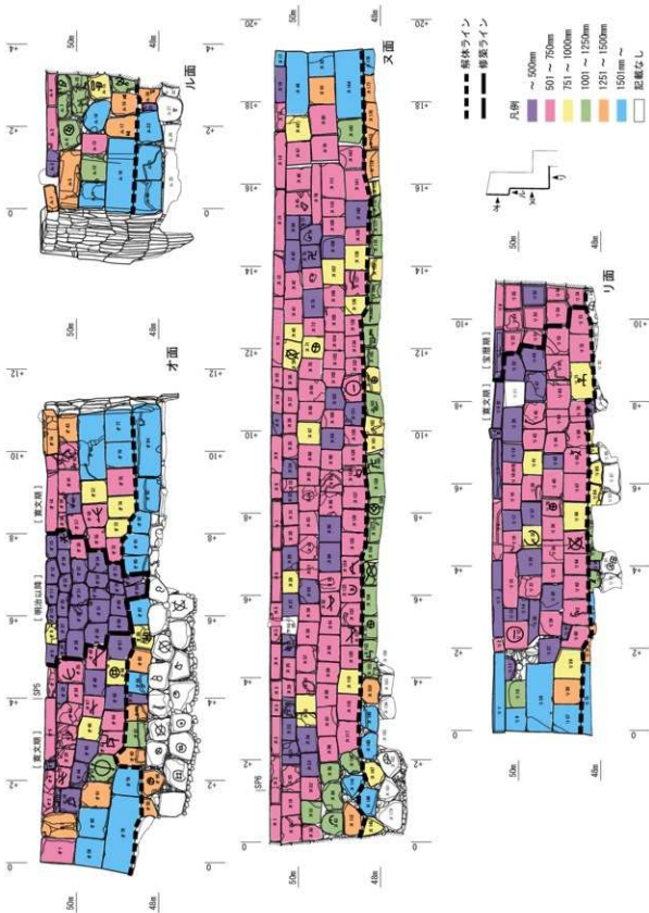
第170図 控え長別色分け図3 才 (2140W)・ル (2140S)・ス (2130W)・又 (2130S) (S=1/100)
