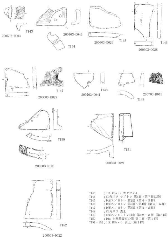
第165図 出土遺物実測図 瓦20 (いぶし・軸, S=1/6)
