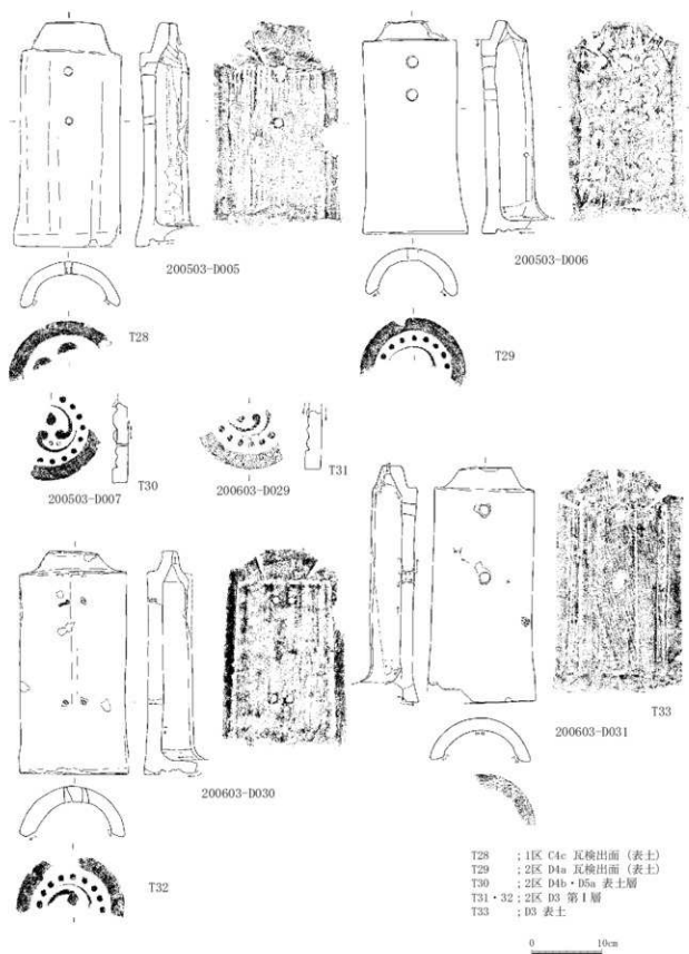
第149图 出土遺物実測图 瓦4 (袖菜, S=1/6)
