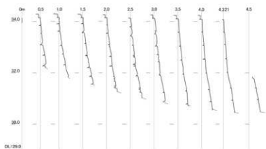
玉泉院丸南西石垣 解体修復後 断面図(垂直) (E面)
