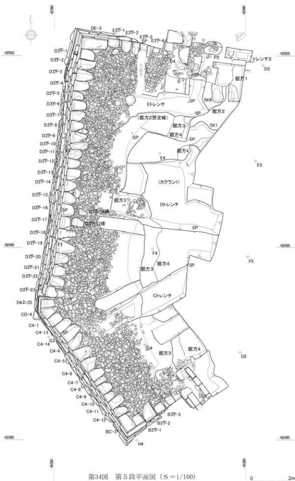
第34図 第5段平面図 (S=1/100)
