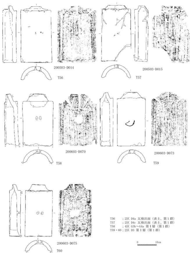
第153图 出土遺物実測图 瓦 8 (袖菜, S=1/6)
