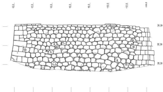
玉泉院丸南西石垣 解体調査修復後 立面図 (E面)
