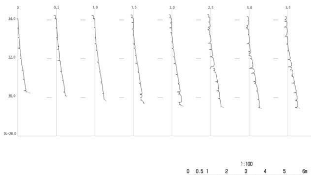
第207図 修復後石垣垂直断面図2
