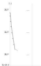
玉泉院丸南西石垣 解体調査修復後 断面図（垂直）（C面）2/2
