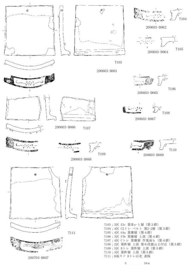
第158図 出土遺物実測図 瓦13 (釉薬, S=1/6)
