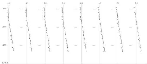
玉泉院丸南西石垣 解体調査修復後 断面図（垂直）（D面）2/4
