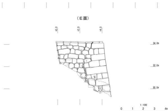
第2図 石垣立面図2
