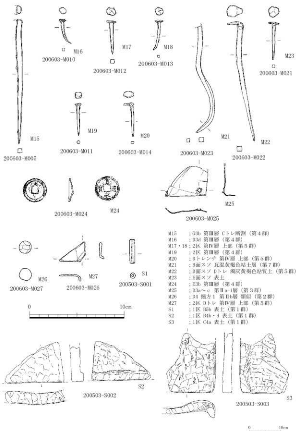
第173図 出土遺物実測図 金属2・石製品 (S=1/2、1/6)
