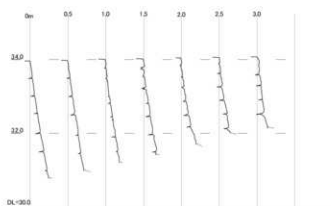
玉泉院丸南西石垣 解体修復後 断面図(垂直) (B面)
