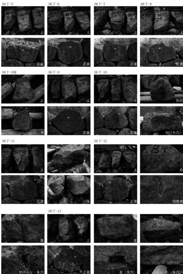
第132図 石材観察写真37 第11段-2
