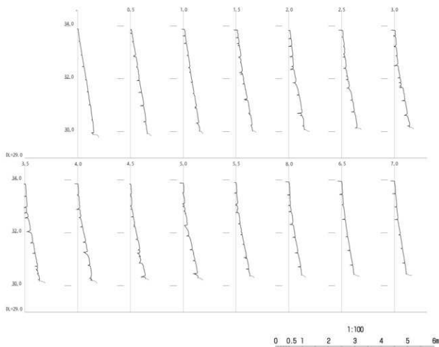
第206図 修復後石垣垂直断面図 1
