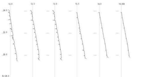
玉泉院丸南西石垣 解体調査修復後 断面図(垂直) (D面) 4/4
