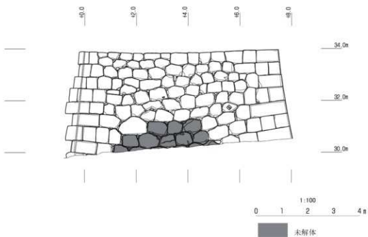
第198図 修復後石垣立面図1
