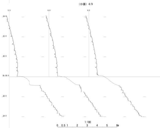
第18图 石坝垂直断面图 4
