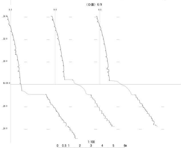
第19图 石垣垂直断面图5
