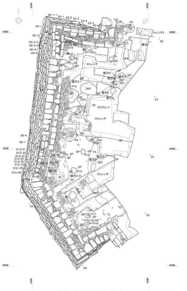
第22図 第0段平面図 (S=1/100)
