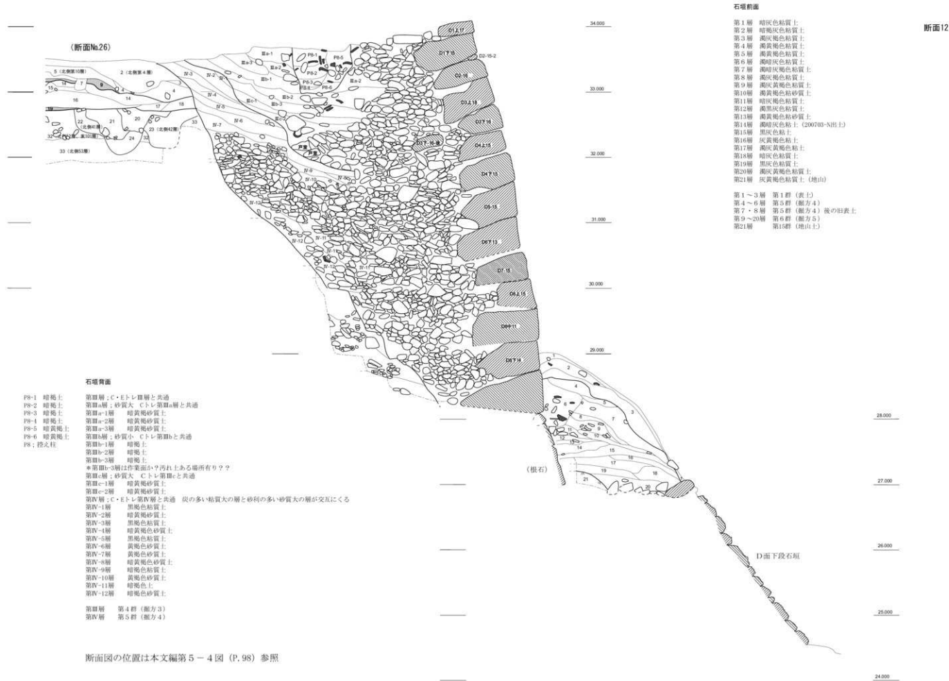
第69図 断面No.12 Dトレンチ土層断面南壁 (S=1/40)
