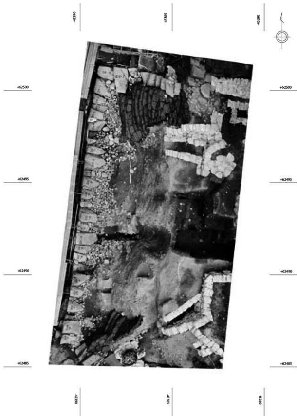
第59图 第16-1段平面写真 (S=1/100)
