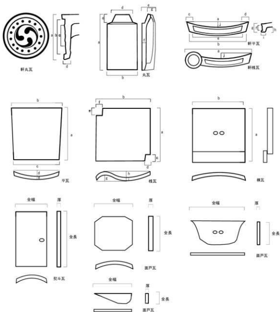
軒丸瓦(軒部) a 瓦当径 b 文様区径 c 内区径 d 瓦当厚 軒平瓦・軒棧瓦 a 上弧幅 b 下幅 c 右側縁 d 左側縁 e 文様区幅 (軒部・平部) f 文様区厚 g 瓦当厚 h 弧高 i 顎下部厚 j 弧深 丸瓦 a 全長 b 体部幅 c 瓦縁長 d 瓦縁高 e 体部高 f 体部厚 g 瓦縁高 平瓦 a 全長 b 瓦端幅 c 瓦端幅 d 瓦端厚 e 厚 棧瓦 a 全長 b 全幅 c 平部切込長 d 平部切込幅 e 棧部切込長 f 棧部切込幅 g 棧部弧深 h 平部弧深 i 厚
