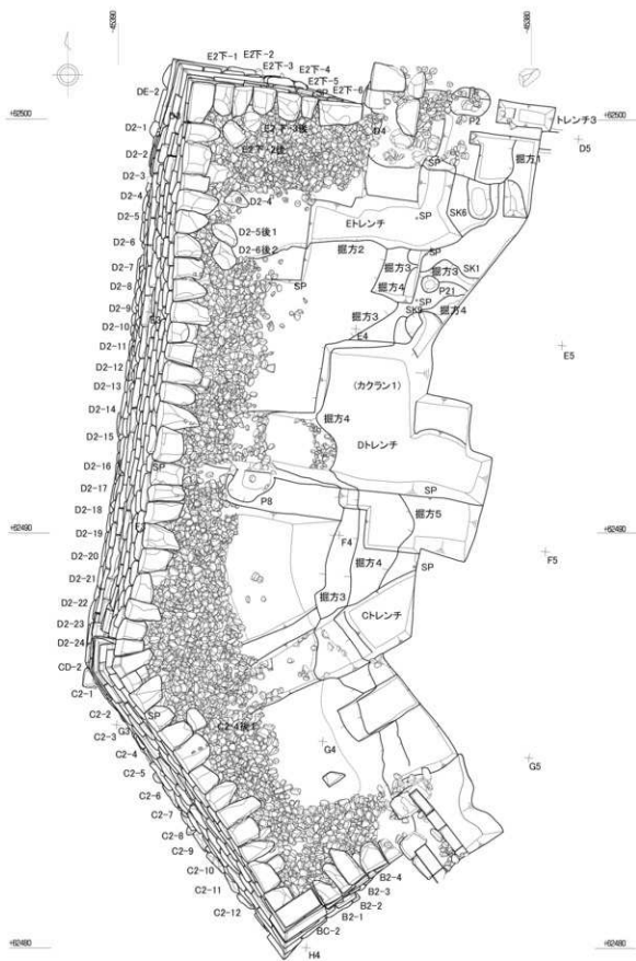
第30図 第3段平面図 (S=1/100)
