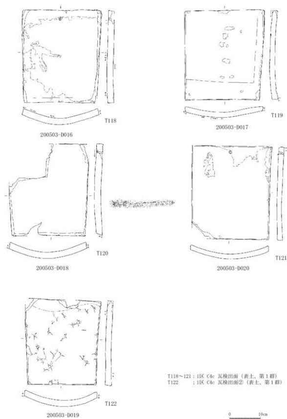
第160図 出土遺物実測図 瓦15 (袖菜, S=1/6)
