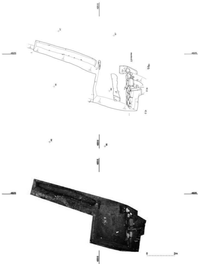
第74图 北拉张区平面图·平面写真(S=1/80)
