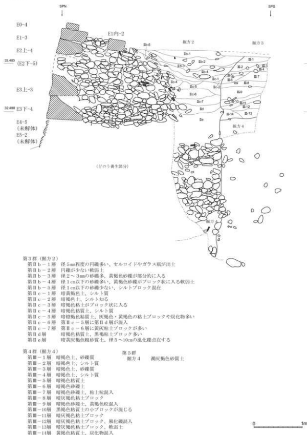
第72図 断面No.17 Eトレンチ土層断面図2 (S=1/40)
