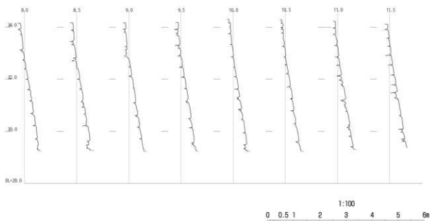
玉泉院丸南西石垣 解体調査修復後 断面図（垂直）（D面）3/4
