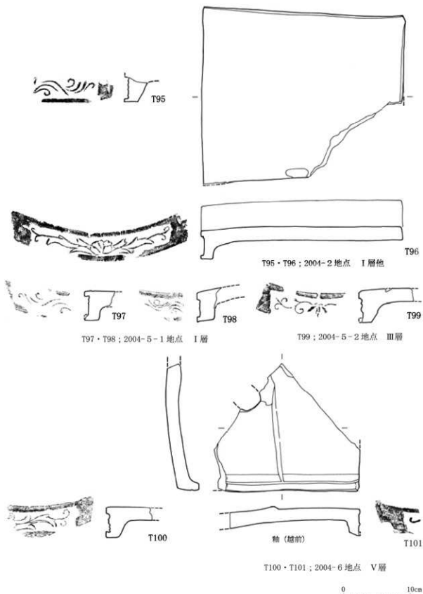
第135図 出土遺物実測図 瓦 (10) (S=1/4)
