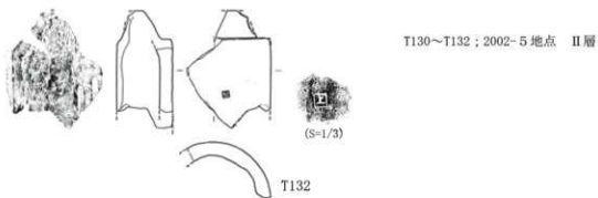
第140図 出土遺物実測図 瓦(15) (S=1/6)
