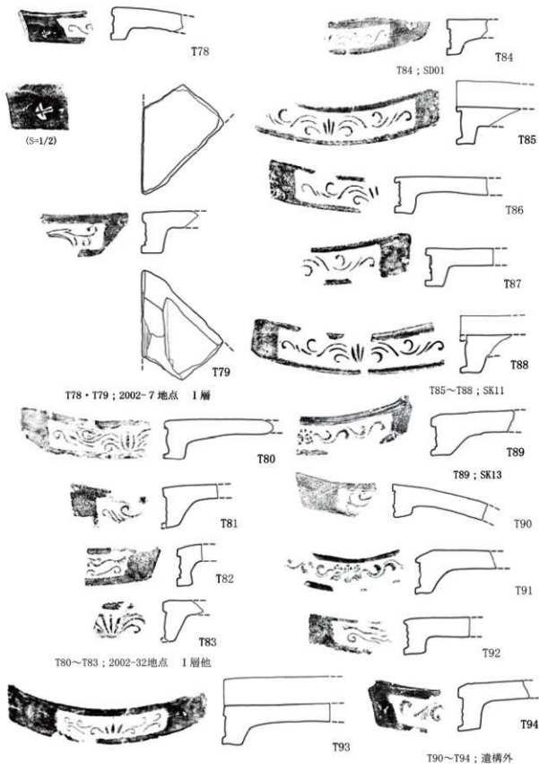
第134図 出土遺物実測図 瓦(9) (S=1/4)
