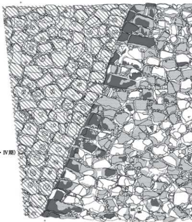
(本丸申西櫓下石垣 粗加工石積み石垣Ⅲa類 石垣編年2期前半 慶長前期)
