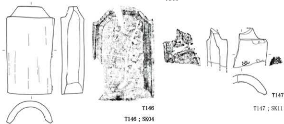
第143图 出土遺物実測図 瓦 (18) (S=1/6)
