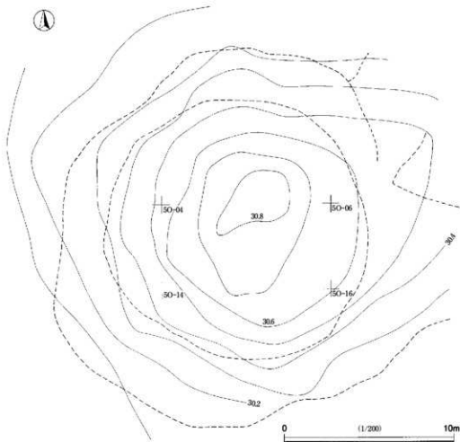
第23図 S19号墳墳丘図
