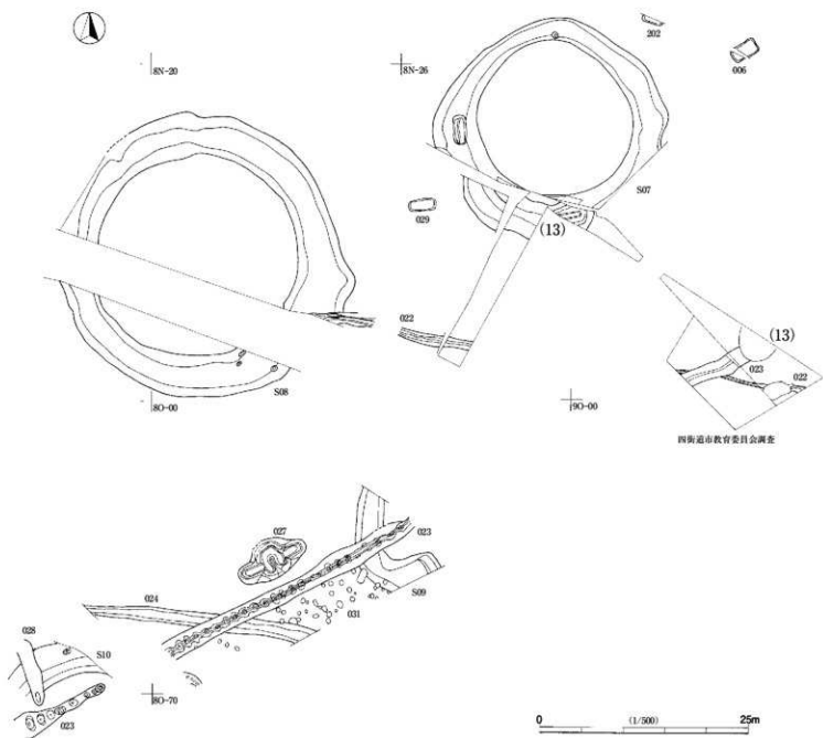
第 9 図 遺構分布図 (1)
