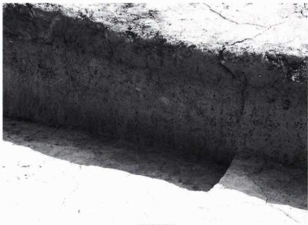
3区東壁断面
