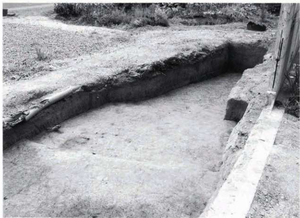
4区東壁断面
