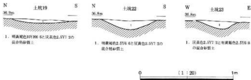
図13 丹上遺跡土坑断面図 (1:20)
