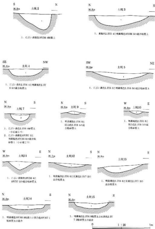
図11 丹上遺跡土坑断面図 (1:20)
