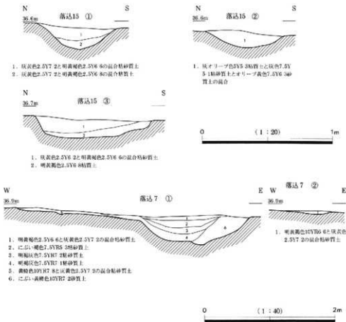
図16 丹上遺跡落込断面図 (1:20, 1:40)
