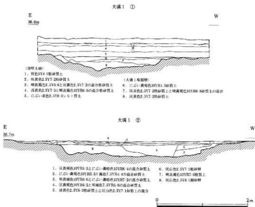
図9 丹上遺跡大溝1断面図(1:40)
