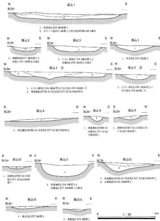
図15 丹上遺跡落込断面図 (1:20)
