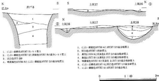
図12 丹上遺跡土坑、井戸断面図 (1:40)
