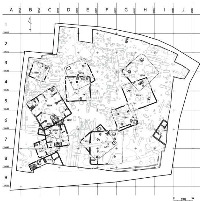
第 12 図 古墳時代遺構分布図 (1 / 300)
