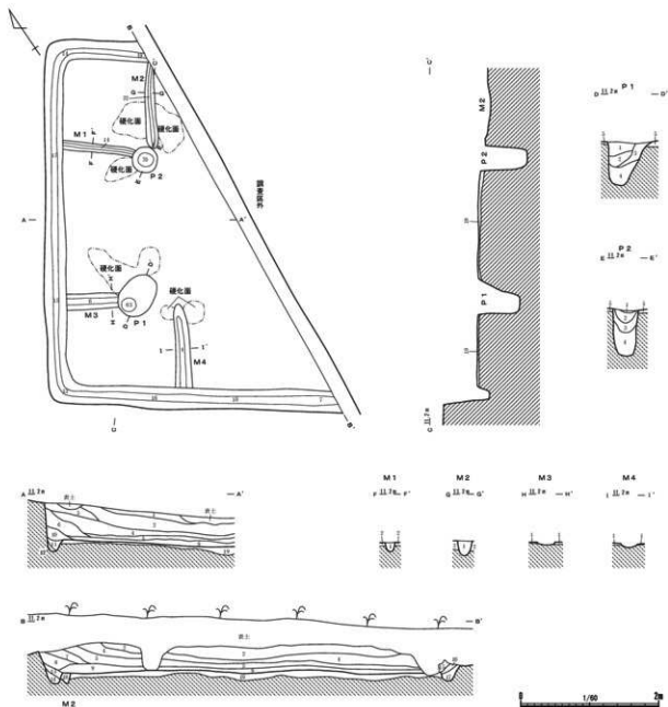
第13図 324号住居跡 (1/60)
