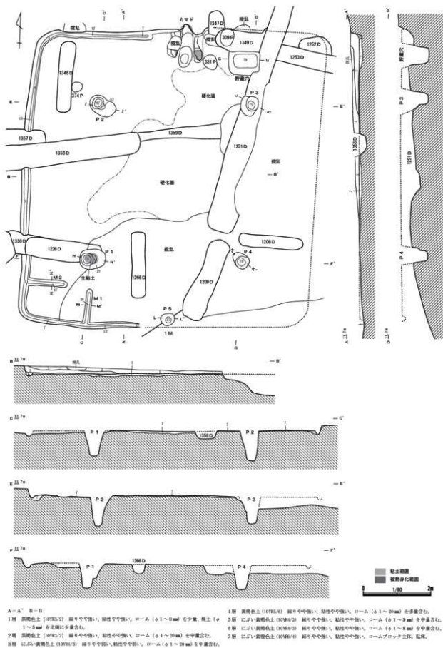
第27図 329号住居跡 (1/80)
