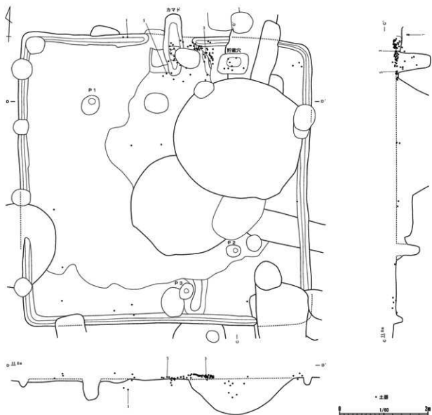
第52図 334号住居跡・遺物出土状態 (1/60)
