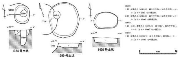
第79図 C群 円形・楕円形の土坑2 (1/60)
