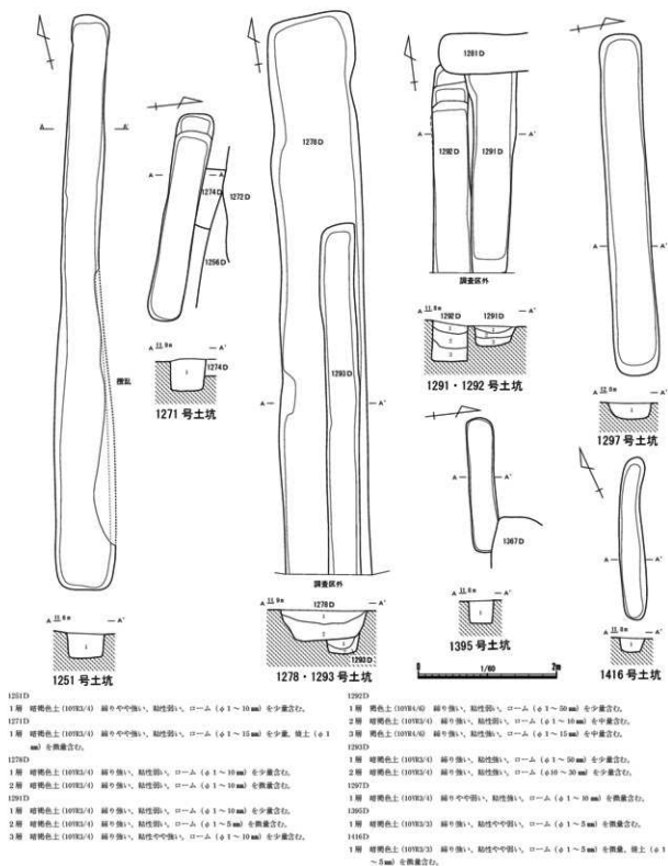
第73図 B群1類 溝状の土坑 (1/60)
