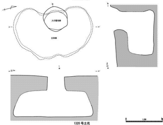
第84図 E群1類 地下室・地下坑(単一主体部) 2 (1/60)
