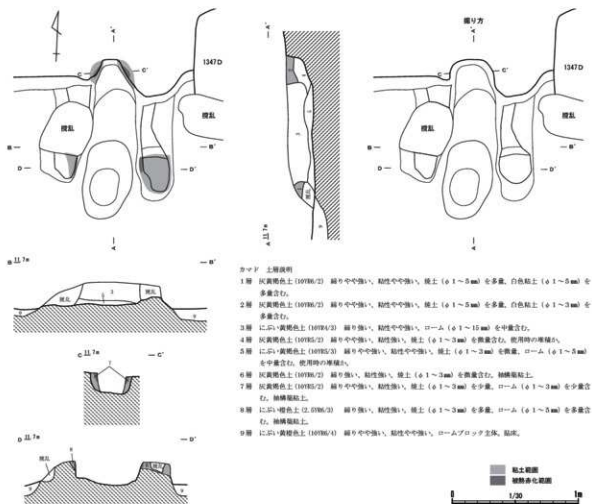
第29図 329号住居跡カマド (1/30)
