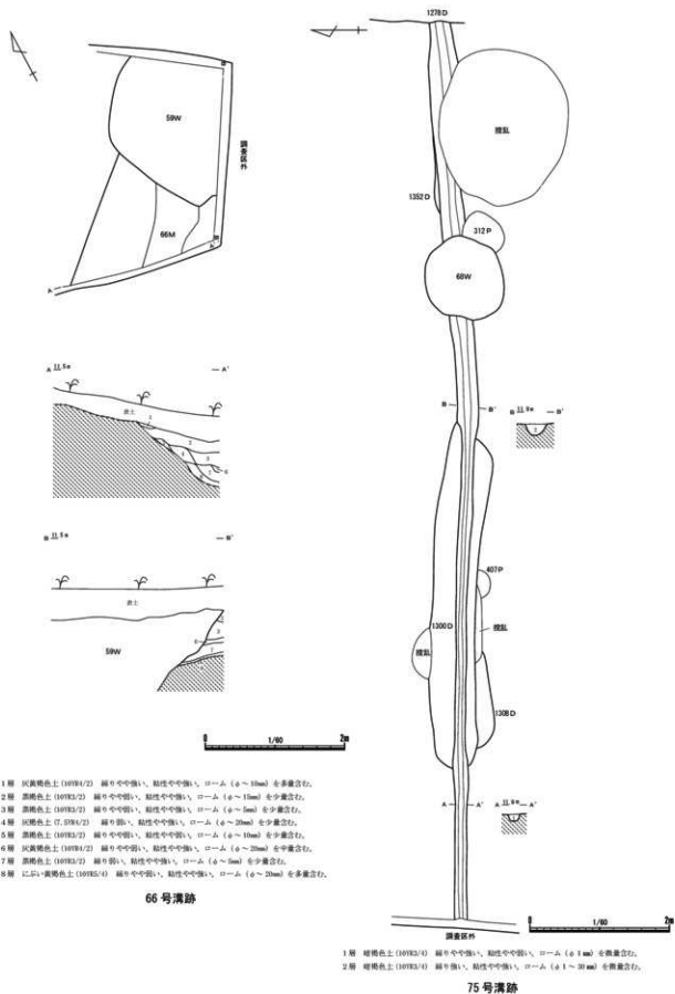
第104図 66・75号溝跡 (1/60)
