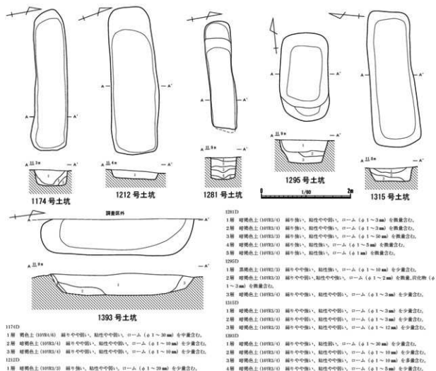
第74図 B群2類 幅狭長方形の土坑 (1/60)
