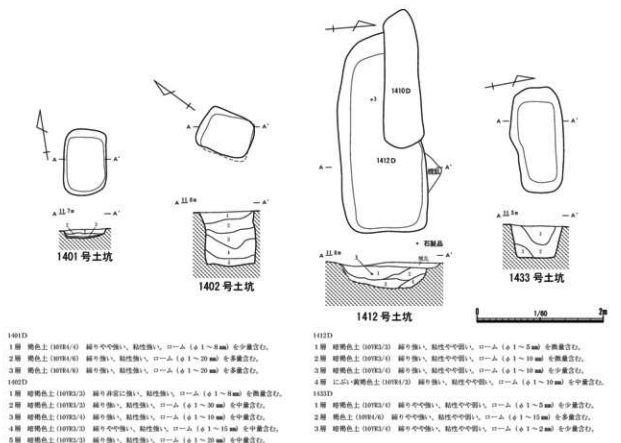
第77図 B群3類 幅広長方形の土坑3 (1/60)
