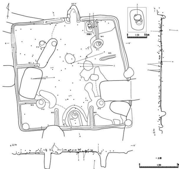
第43図 332号住居跡遺物出土状態(1/60・1/30)
