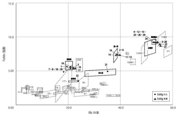
第129図 望月ダイアグラム (Rb 分率図)
