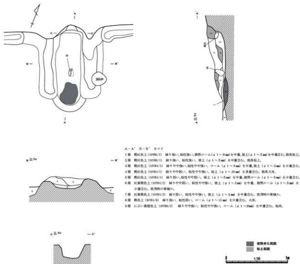
第38図 331号住居跡カマド(1/30)
