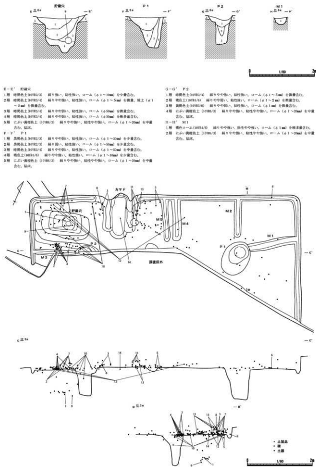
第36図 331号住居跡・遺物出土状態 (1/60)
