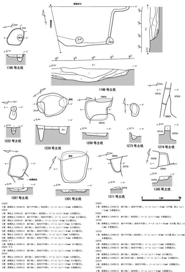
第80図 D群 不整形の土坑1 (1/60)
