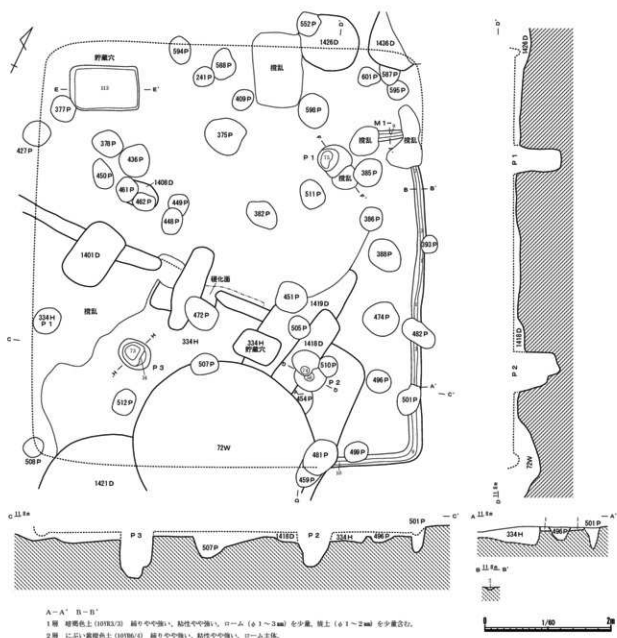
第59図 336号住居跡 (1/60)
