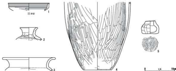
第54図 334号住居跡出土遺物 (1/4)
