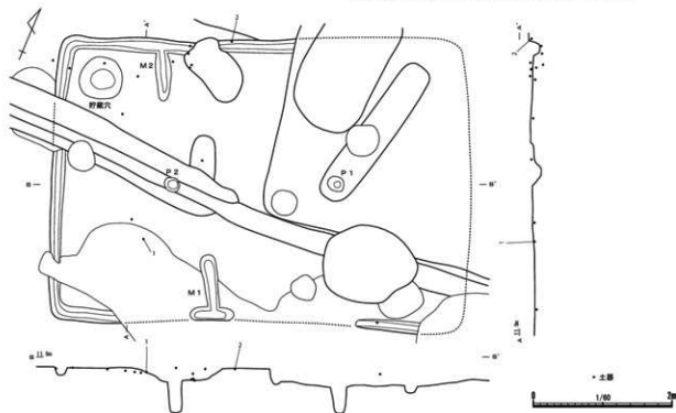
第25図 328号住居跡・遺物出土状態 (1/60)
