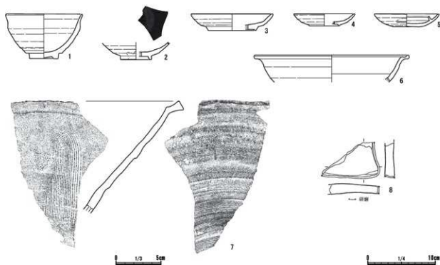
第102図 1号溝跡出土遺物(1/3・1/4)
