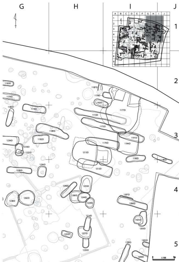
第91图 土坑区分图3 (1/100)
