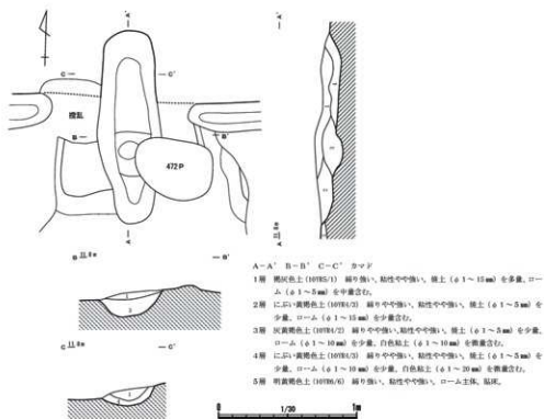
第53図 334号住居跡カマド (1/30)
