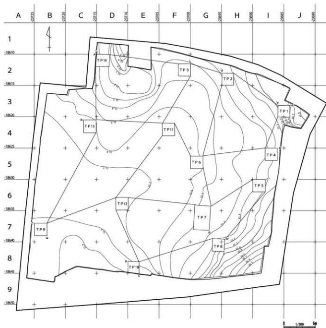
第5図 基本層序の位置 (1/300)
