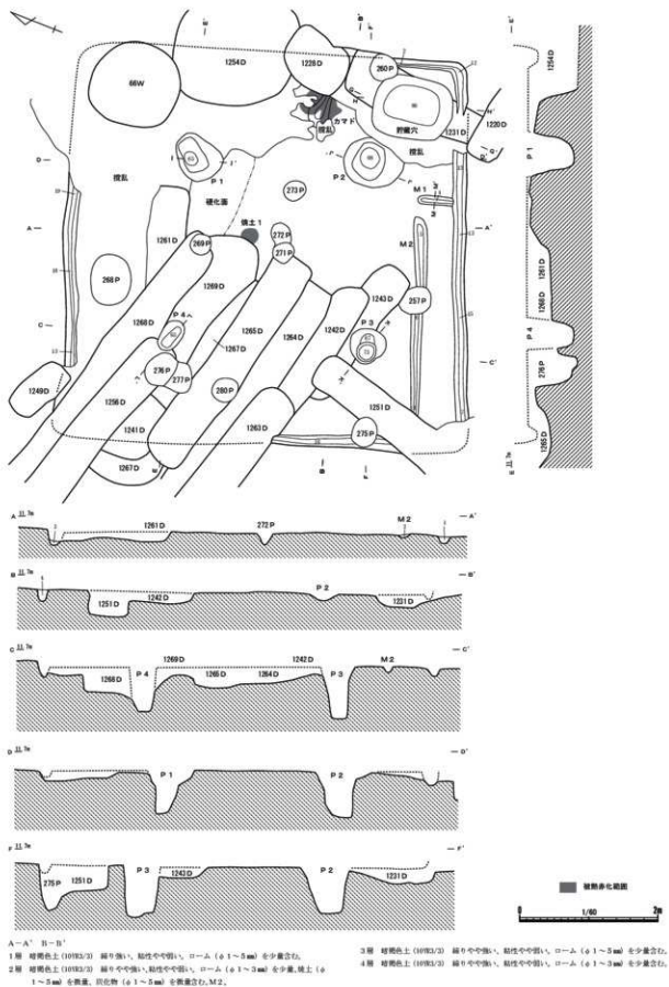
第16図 325号住居跡 (1/60)
