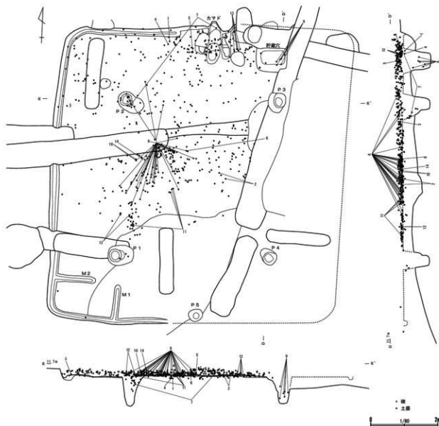
第28図 329号住居跡・遺物出土状態(1/80)
