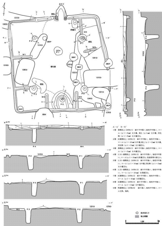
第41図 332号住居跡1 (1/60)
