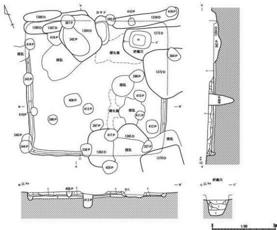
第47図 333号住居跡(1/60)
