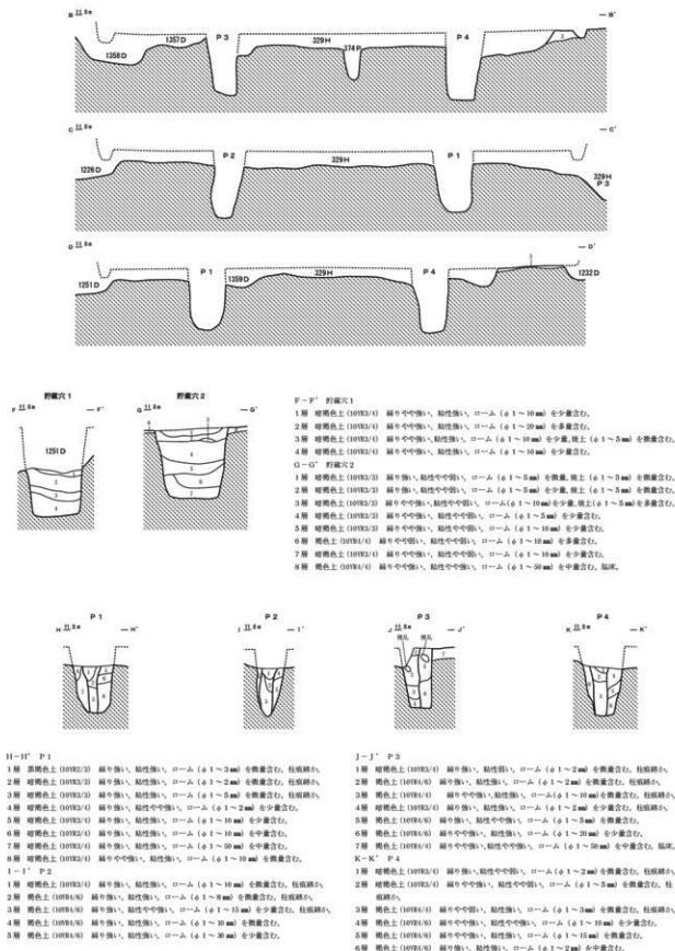
第32図 330号住居跡2 (1/60)
