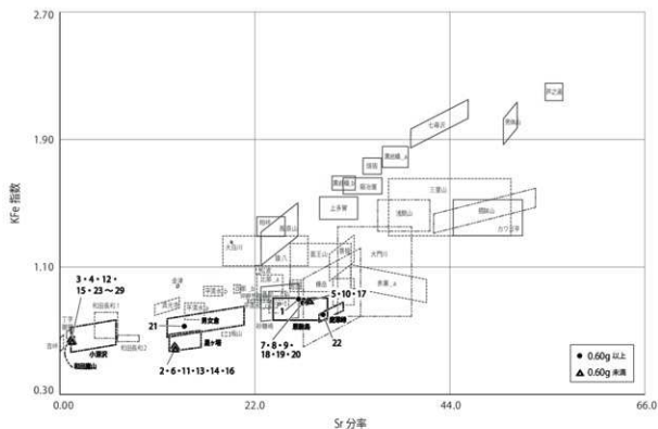
第130図 望月ダイアグラム (Sr 分率図)
