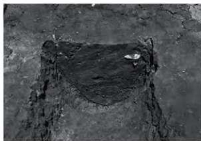
SD11 B断面 (南から)
