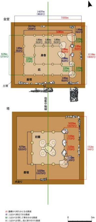
図40 塔と金堂の寸法復元 (1/200)
