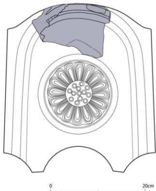
図 33 A種蓮華文鬼瓦の復元案 (1/4)
