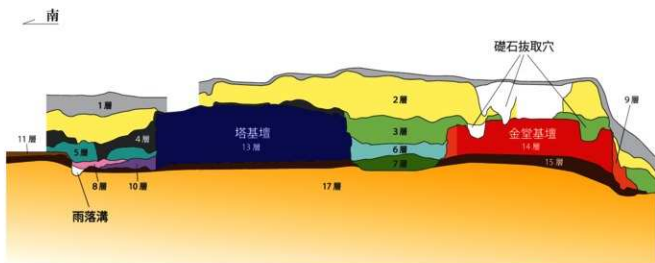
図7 基本層序模式図（縮尺及び縦横比率任意）
