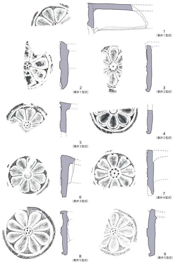
図 26 軒丸瓦実測図 (1/4)
