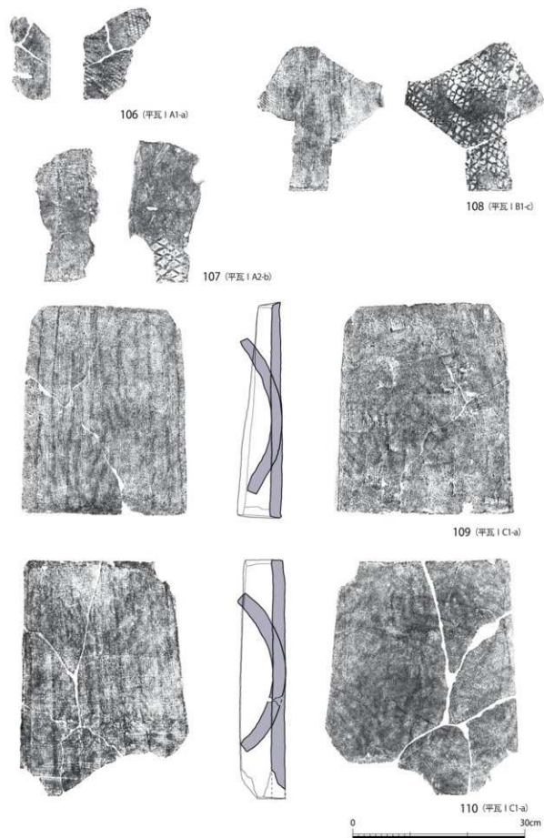
図31 桶巻き作り平瓦実測図 (1/6)
