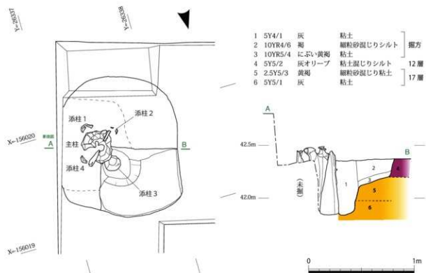
図24 木製灯籠の遺構平面図及び土層断面図 (1/25)
