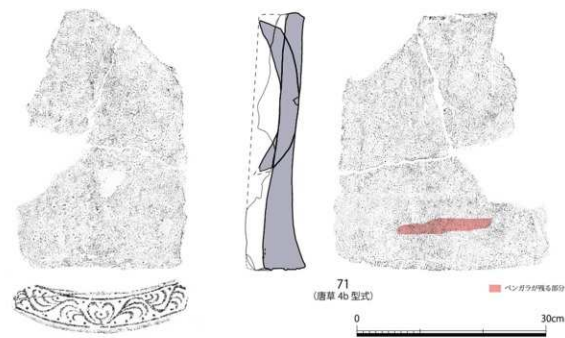
図 27 軒平瓦実測図 (1/6)
