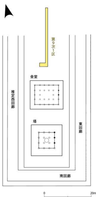
図23 金堂北方の調査位置図 (1/500)
