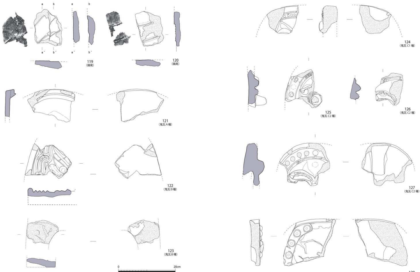
图34 鴟尾・兔瓦实测图(1/4)
