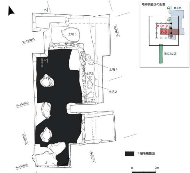
図13 塔4層及び6層上面遺構平面図 (1/100)
