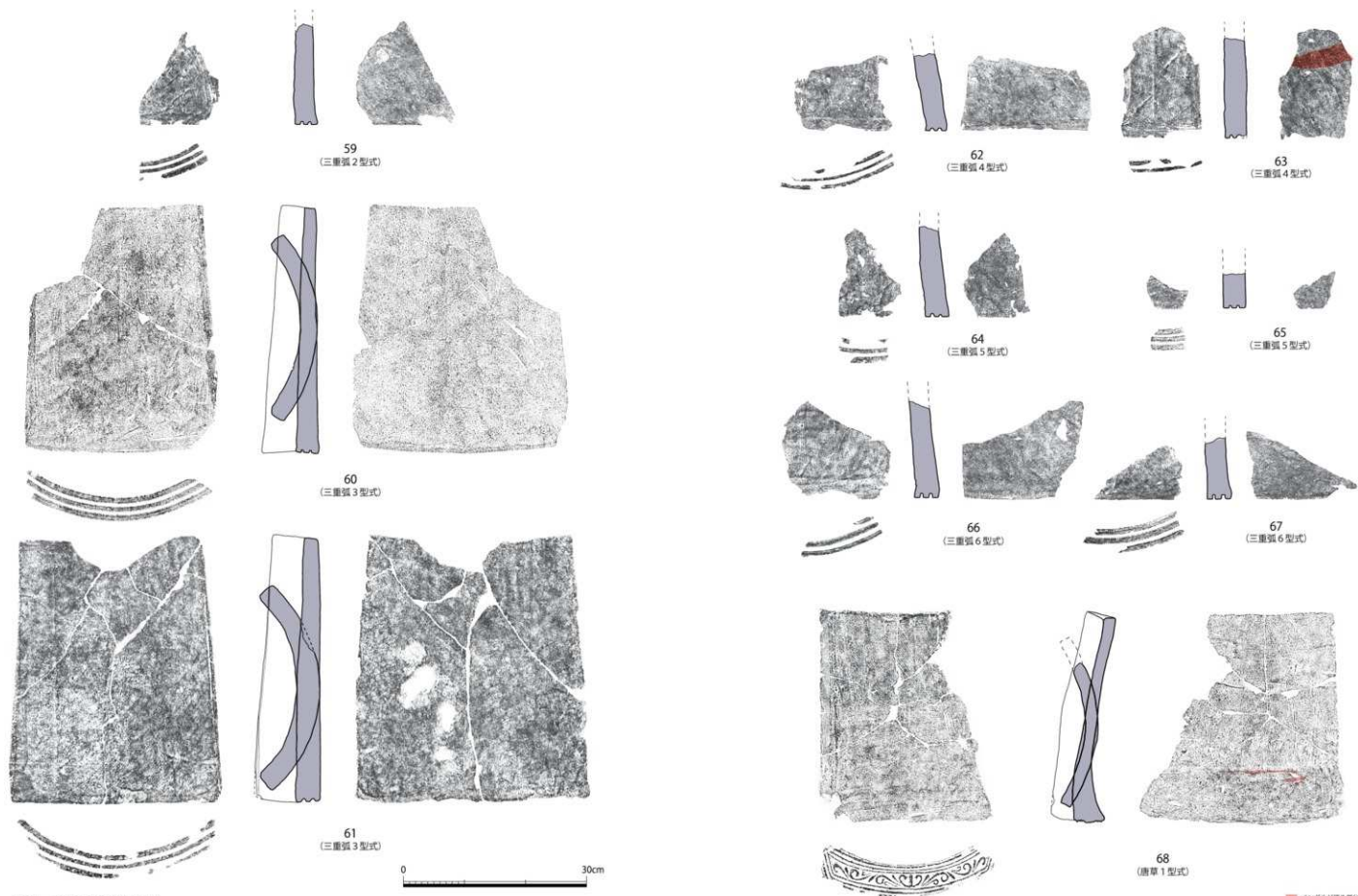
図 27 軒平瓦実測図 (1/6)
