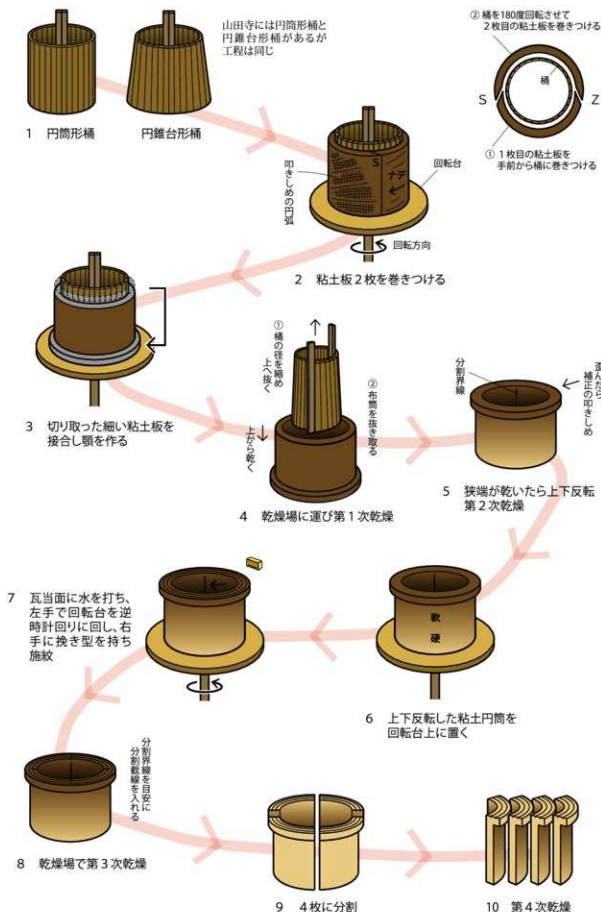
図 47 図解 山田寺出土四重弧紋軒平瓦の製作工程
