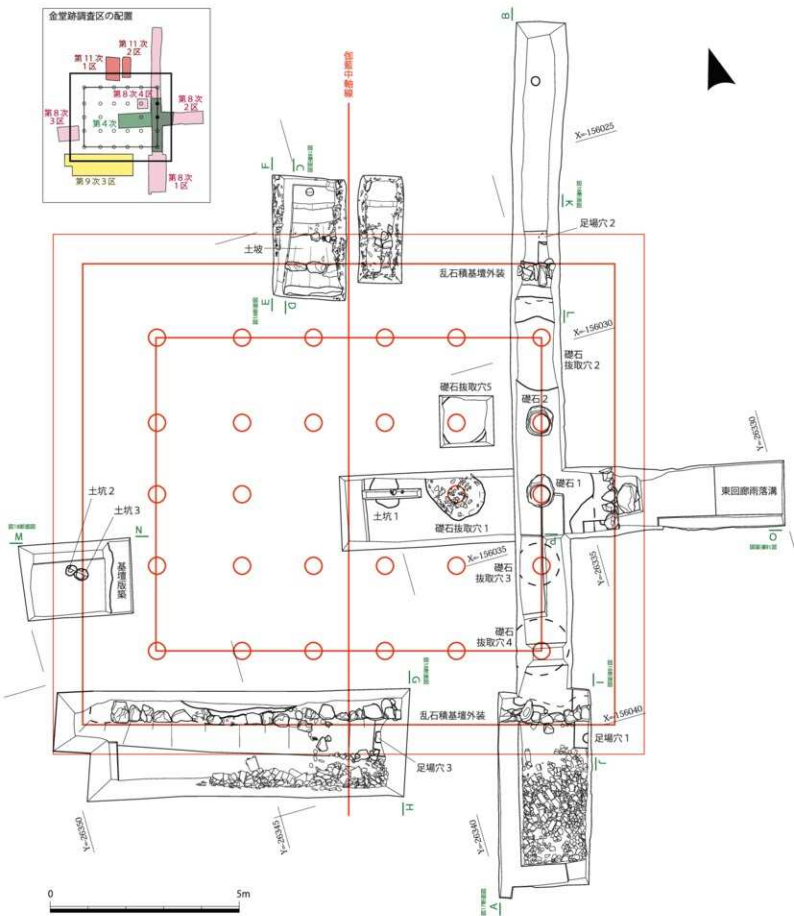
図15 金堂遺構平面図 (1/100)
