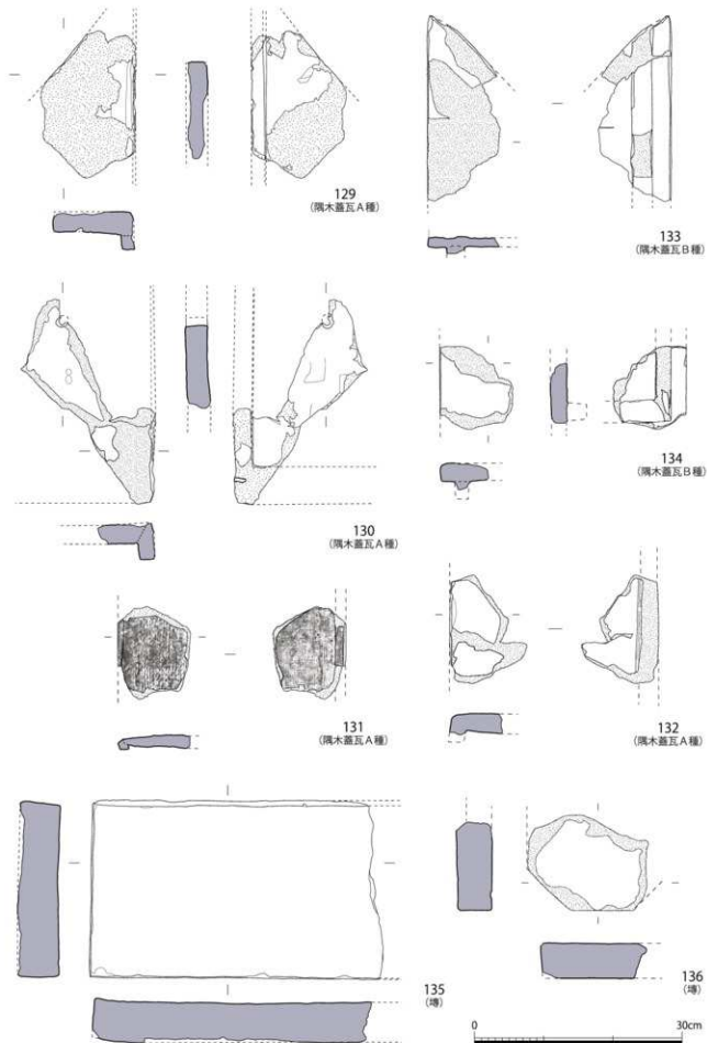
図 35 陶木蓋瓦・埴実測図 (1/6)
