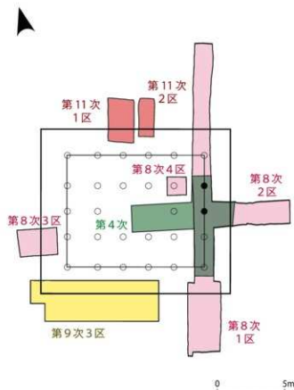
図14 金堂跡調査位置図 (1/250)
