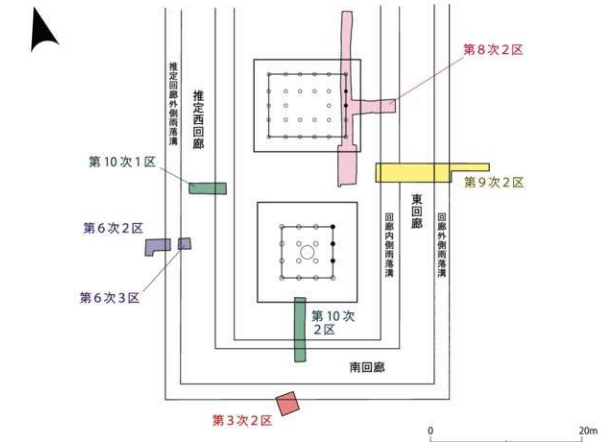
図 20 回廊跡調査位置図 (1/500)
