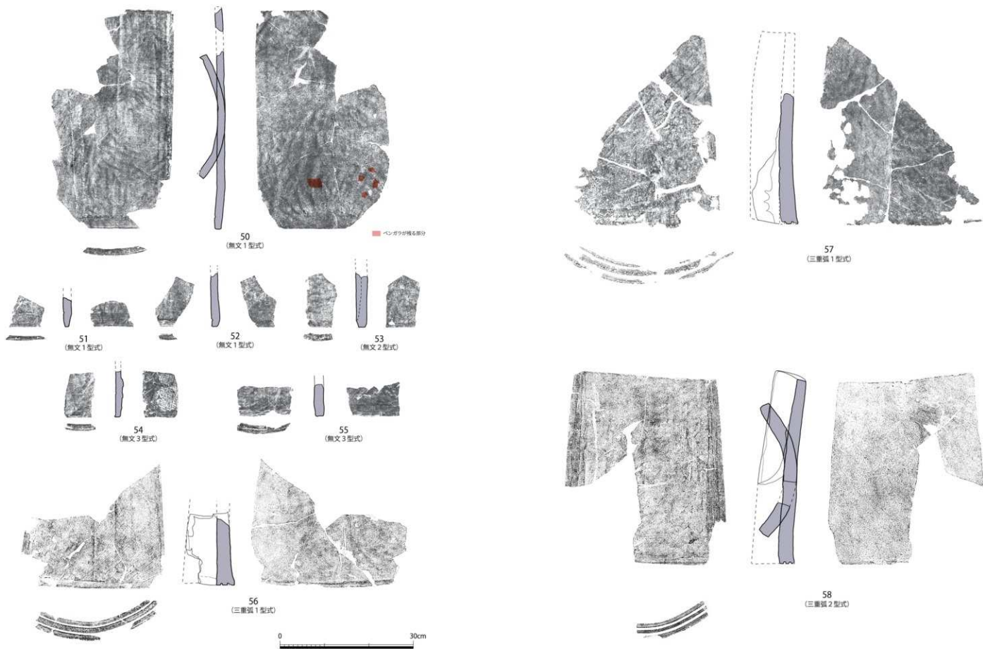
図27 軒平瓦実測図 (1/6)
