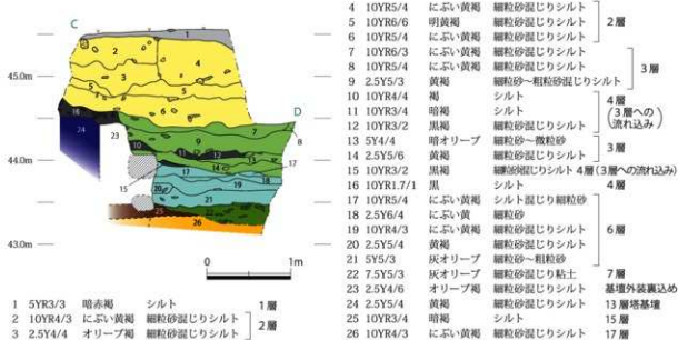
図12 塔北面基壇外周土層断面図 (1/50)
