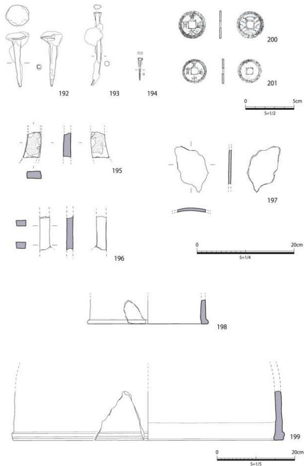
図38 金属製品実測図
