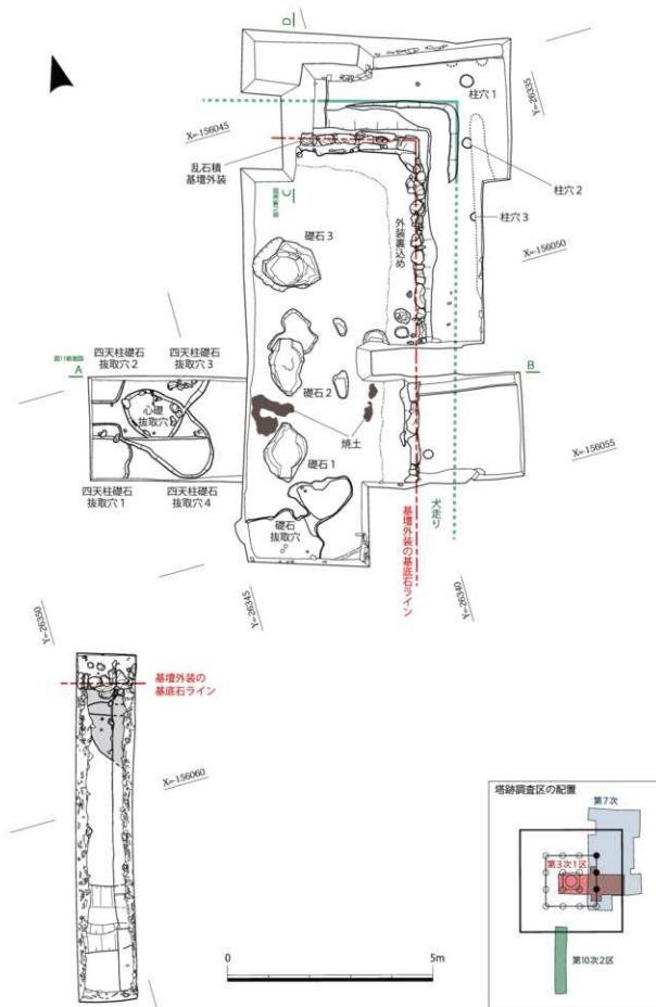
図10 塔遺構平面図 (1/100)
