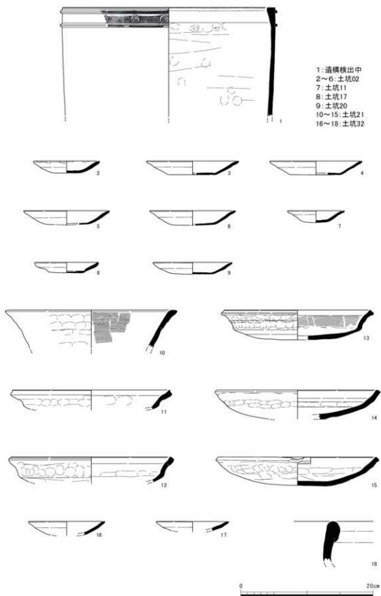
図21 出土遺物 1 (1 : 4)
