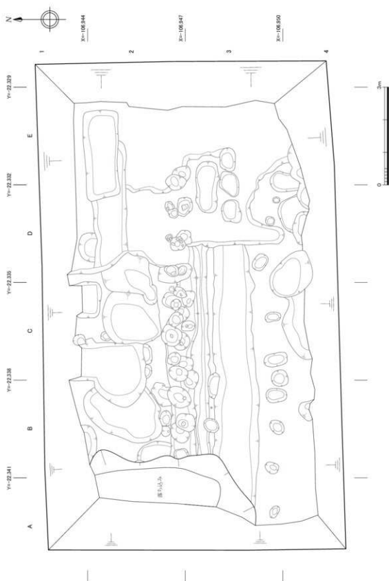
図20 第5層完掘平面図 (1 : 80)
