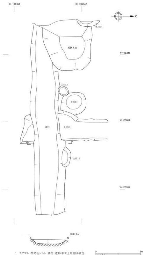
図10 溝13平面・断面図 (1:50)
