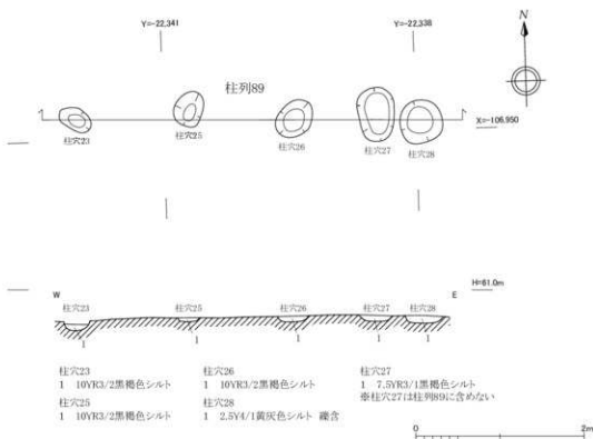
図18 柱列89平面・断面図 (1:50)
