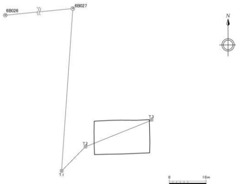
図3 基準点路線図 (1 : 500)
