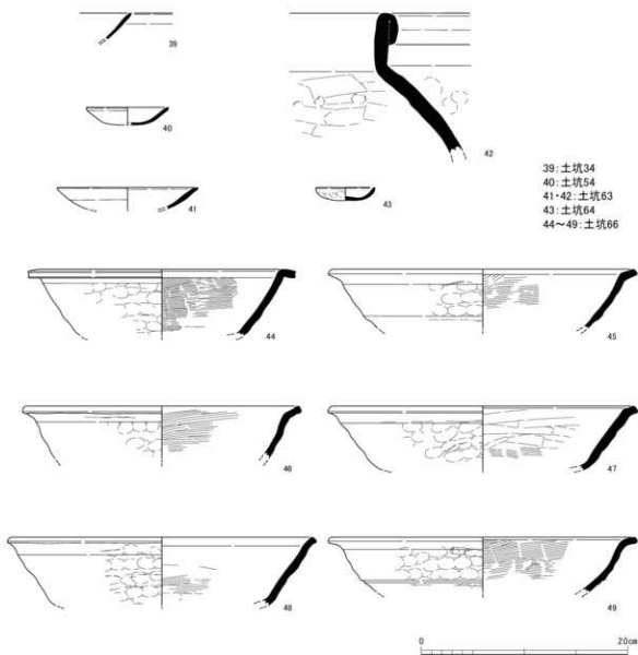
図23 出土遺物3 (1:4)
