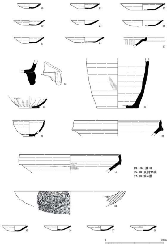
図22 出土遺物 2 (1 : 4)
