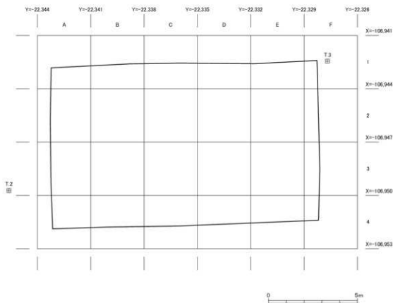
図4 調査区地区割り・基準点配置図 (1 : 150)
