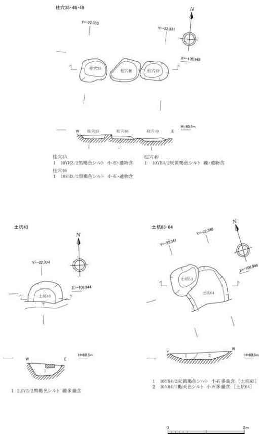
図19 柱穴35・46・49・土坑43・63・64平面・断面図（1：50）
