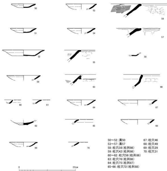
図24 出土遺物4 (1:4)
