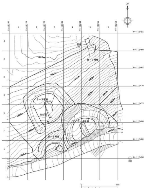
図3 調査区地区割り・基準点配置図 (1:300)
