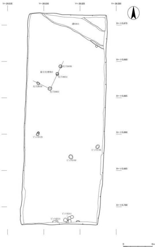
図12 調査区全体平面図（古墳時代）（1：150）
