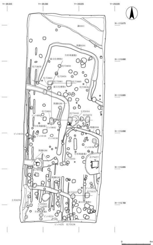
図7 調査区全体平面図 (1 : 150)
