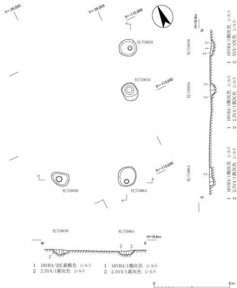
図14 掘立柱建物3 平断面図 (1:50)
