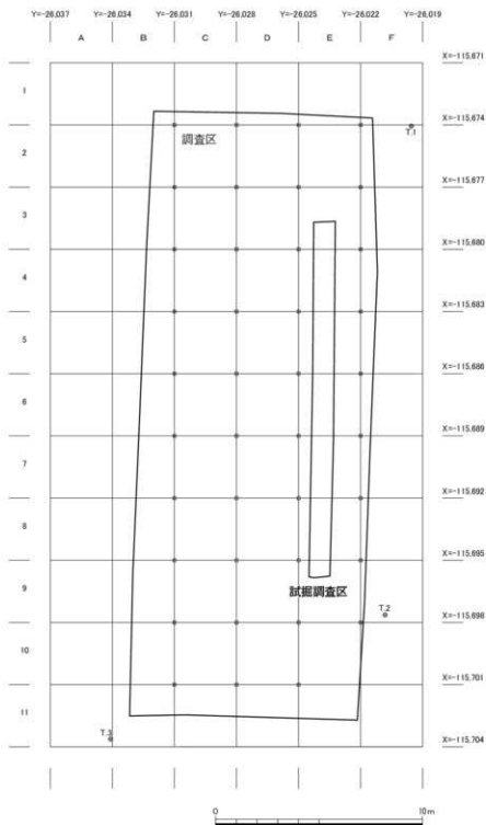
図3 基準点配置、地区割り図 (1 : 200)
