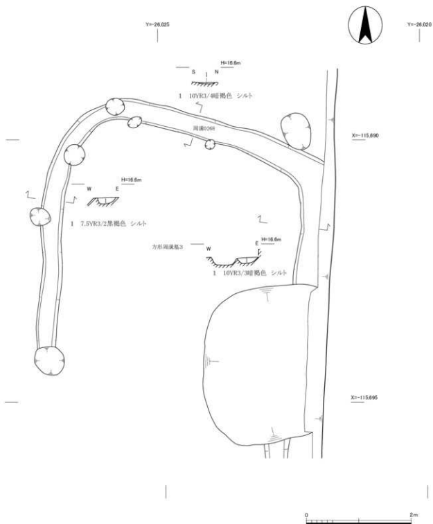
図18 方形周溝墓3平断面図 (1:50)
