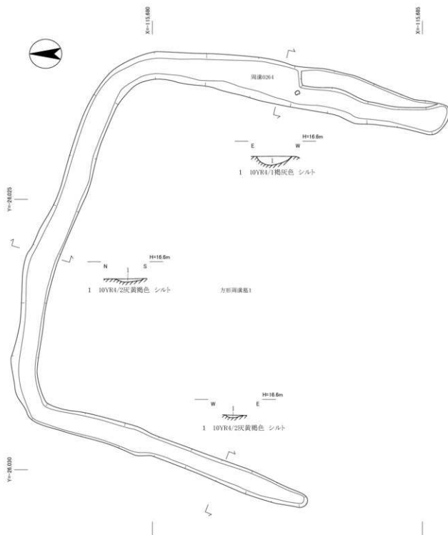
図16 方形周溝墓1平面図 (1:50)
