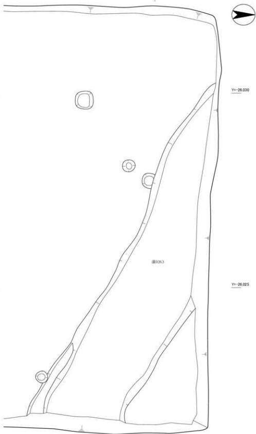
图13 溝0263平面图 (1:50)
