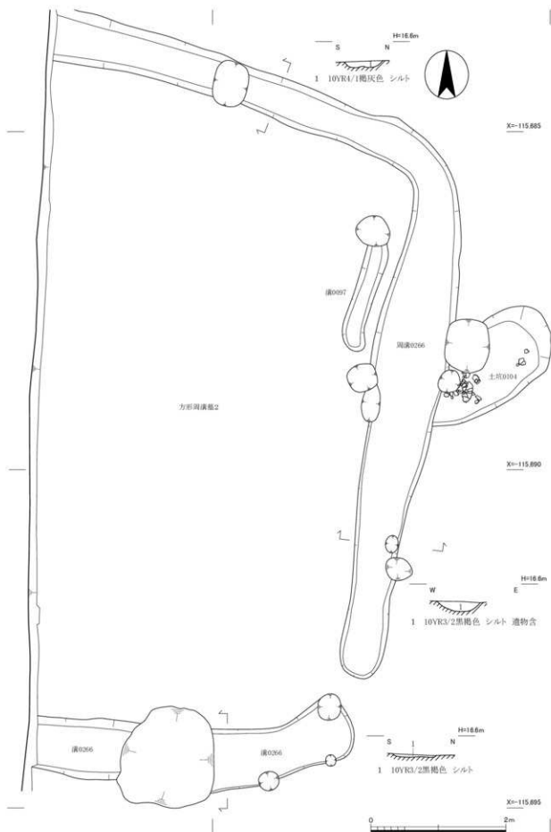
図17 方形周溝墓2平断面図 (1:50)
