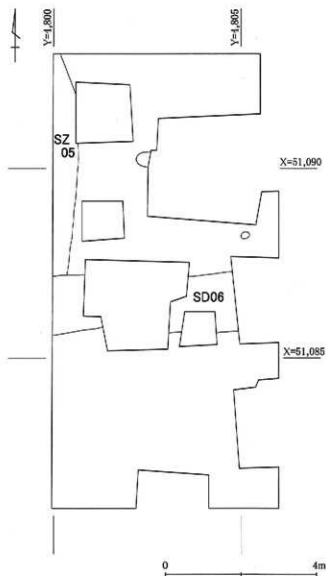
第34図 SB01 東辺延長線上調査区平面図
