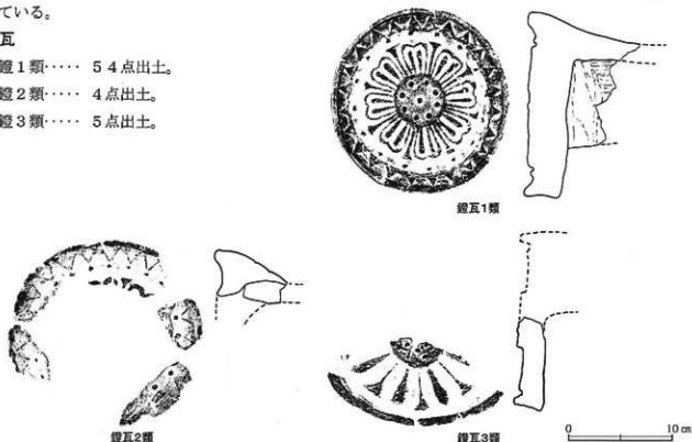
第58図 鏡瓦実測図
