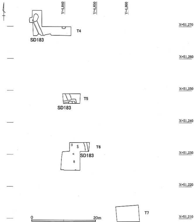
第 40 图 政府東側崖面調査区遺構配置图 (2)
