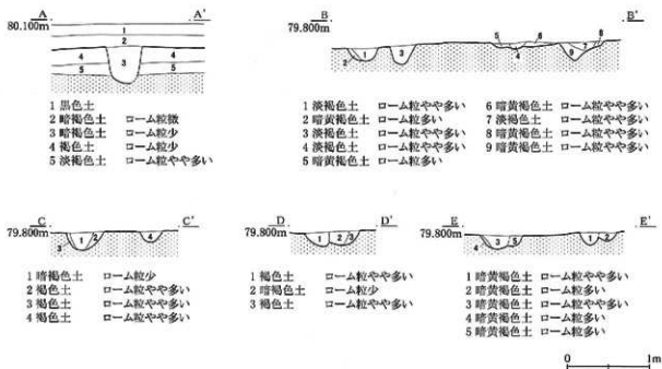
第 55 図 北側範囲確認調査区 T6 (北部) 土層断面図
