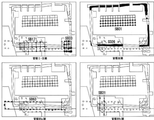
第70図 正倉域中心建物変遷図
