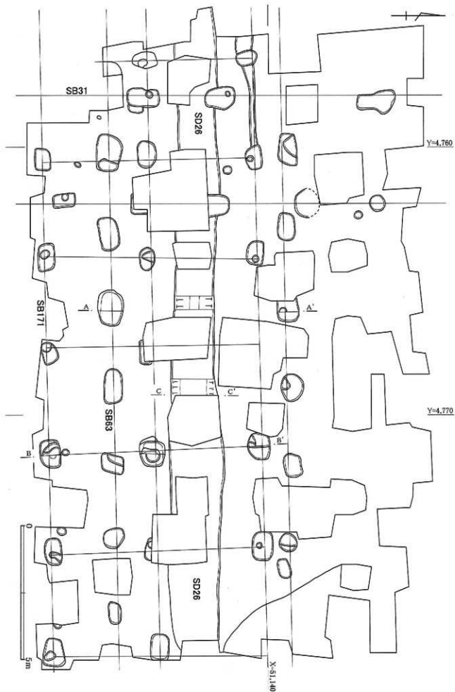
第 21 图 SB01 南侧調査区平面图
