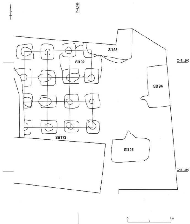
第 27 図 SB173・SI192～195 平面図
