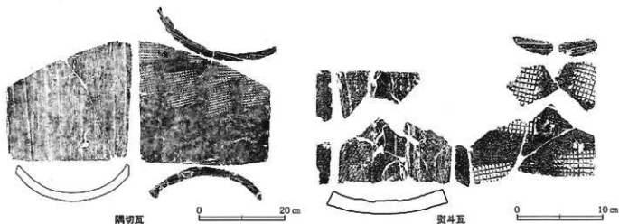
第68図 道具瓦実測図
