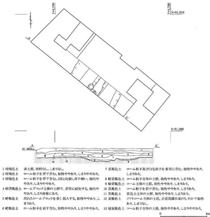
第11図 東山道跡調査区T8平面図・土層断面図
