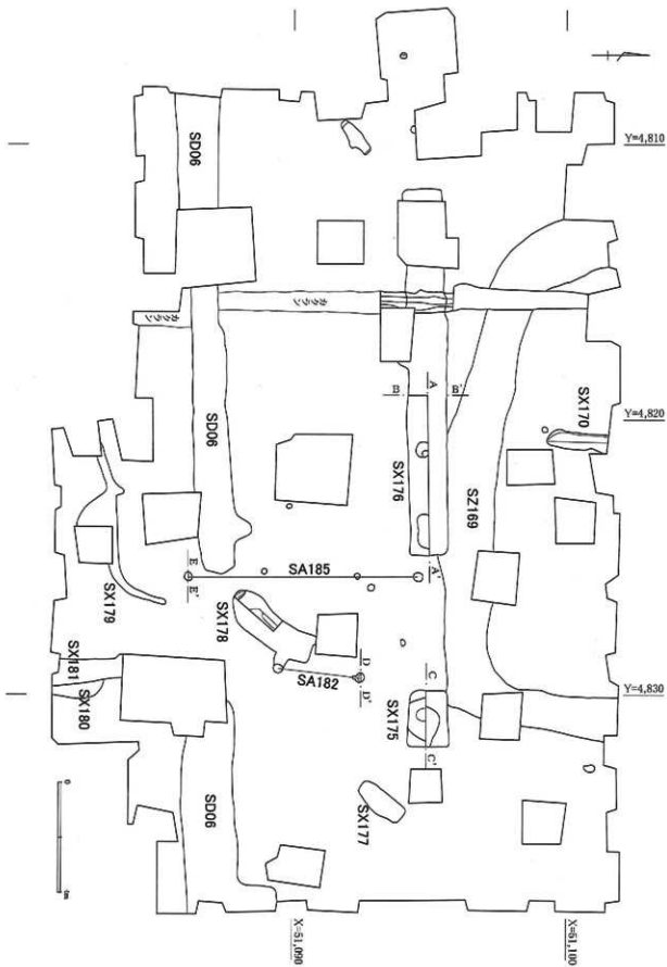
第36图 東側東山道近接部調査区平面图 (1/150)
