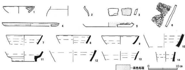
第19図 SB01調査区出土遺物実測図(1)
