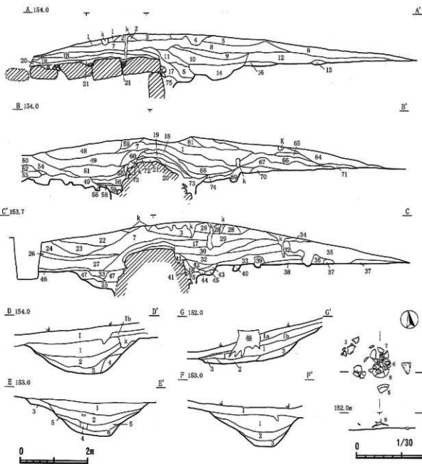
第16図 4号墳丘・周溝土層図
