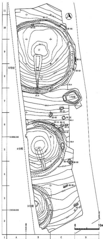
第6図 遺構配置図(1)古墳時代以降
