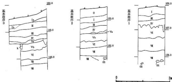
第4図 基本層序
