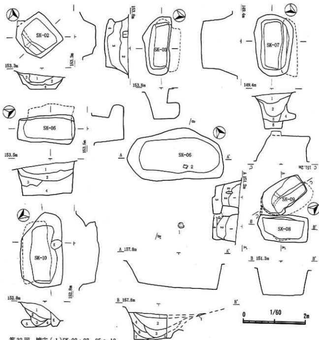
第32図 塚穴(1)SK-02・03、05〜10
