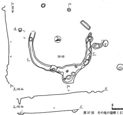
第37図 その他の遺構(2)SX-01・02
