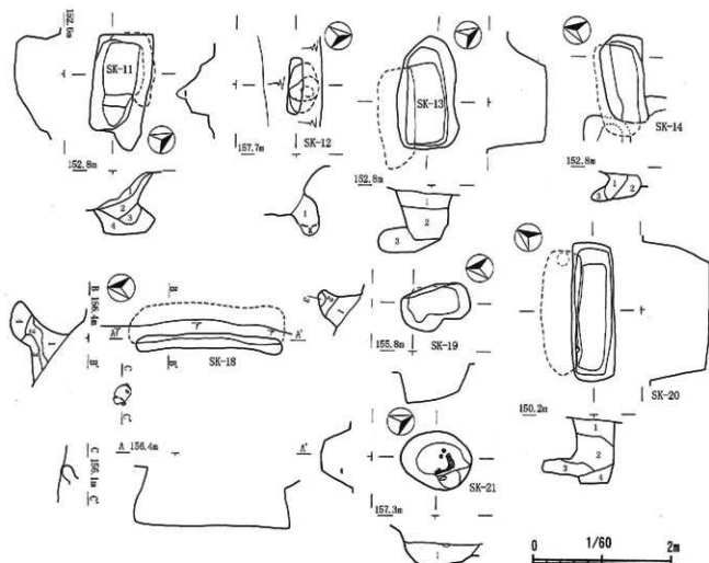
第33図 塚穴(2)SK-11～14、18～21
