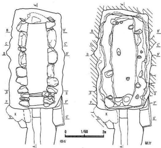
第19図 4号墳石室圖(2)
