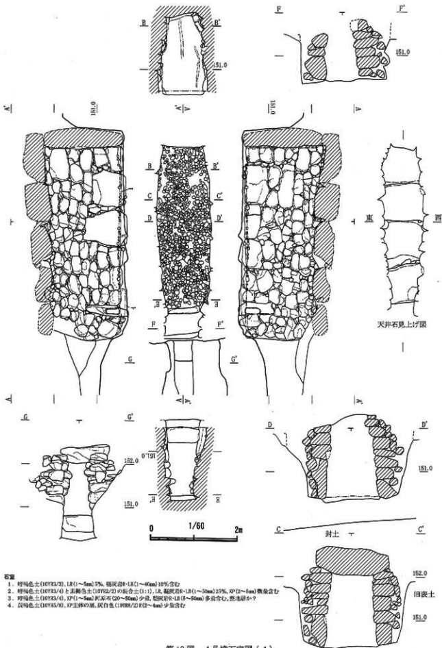
第18図 4号墳石室図(1)
