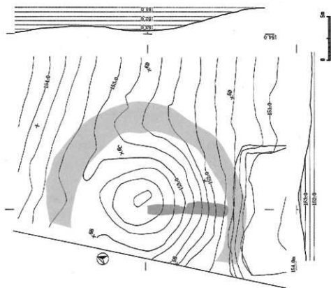
第 14 图 4 号墳现状図
