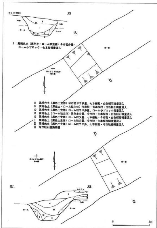
第5図 SD-01実測図(2)
