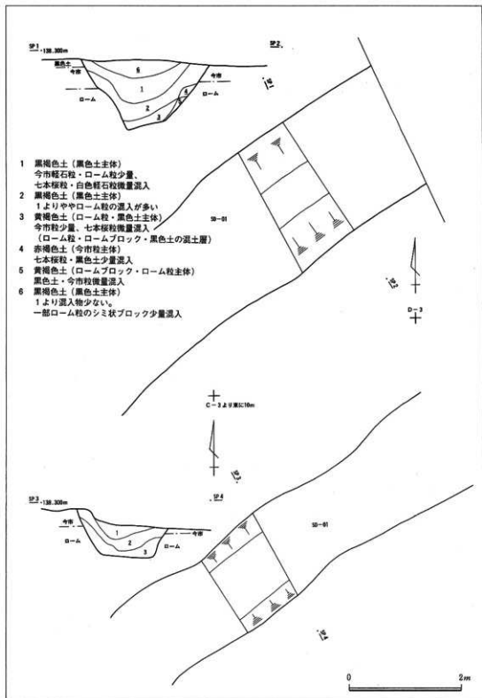
第4図 SD-01実測図(1)
