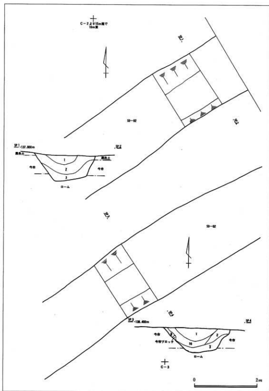
第7図 SD-02実測図(1)
