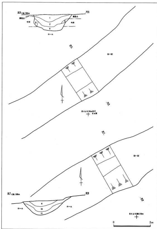
第8図 SD-02実測図(2)
