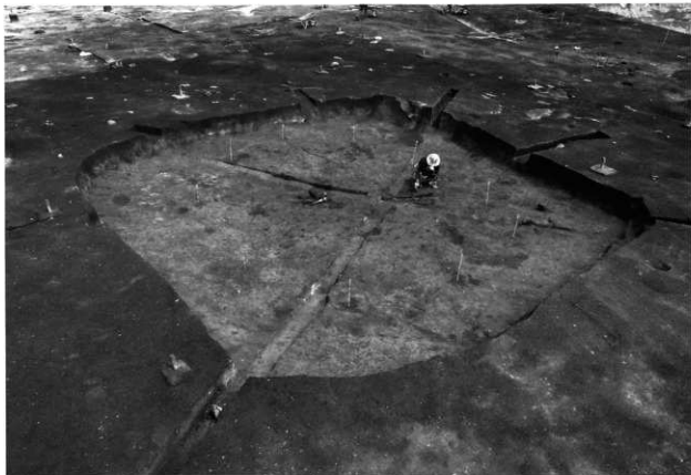
1. VH-07完掘 SW→
