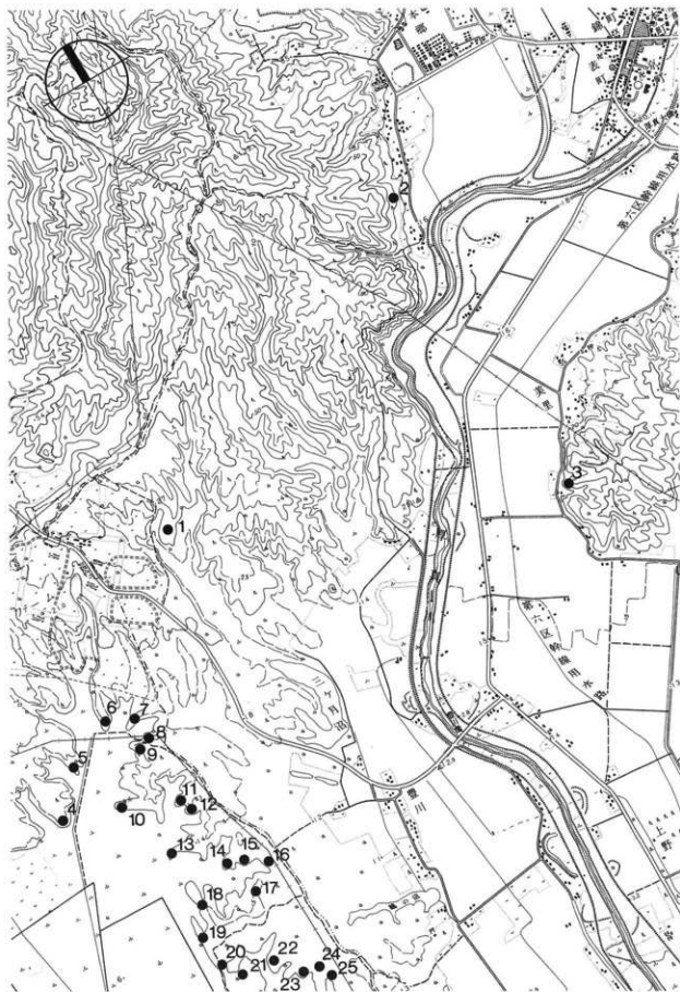
図1 豊川1遺跡と周辺の遺跡 (1/2.5万厚真町管内図を使用)
