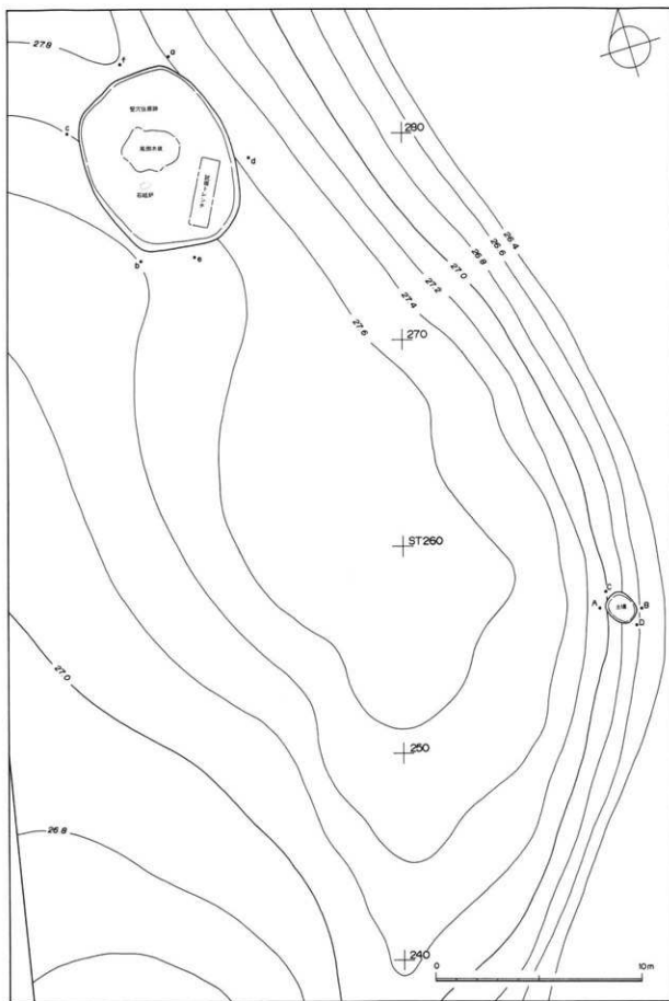
図3 遺構の位置 (コンターはTa-d層上面)
