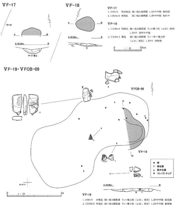
図Ⅲ-10 VF-17~19・VFCB-09 平面及び断面図
