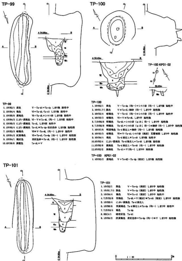
図Ⅲ-13 TP-99～101 平面図及び断面図
