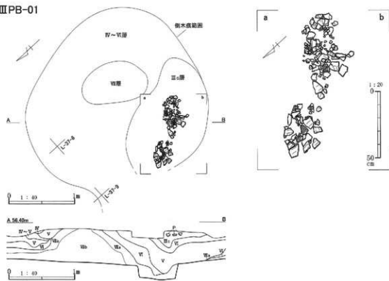
図Ⅱ-3 ⅢPB-01 平面及び断面図
