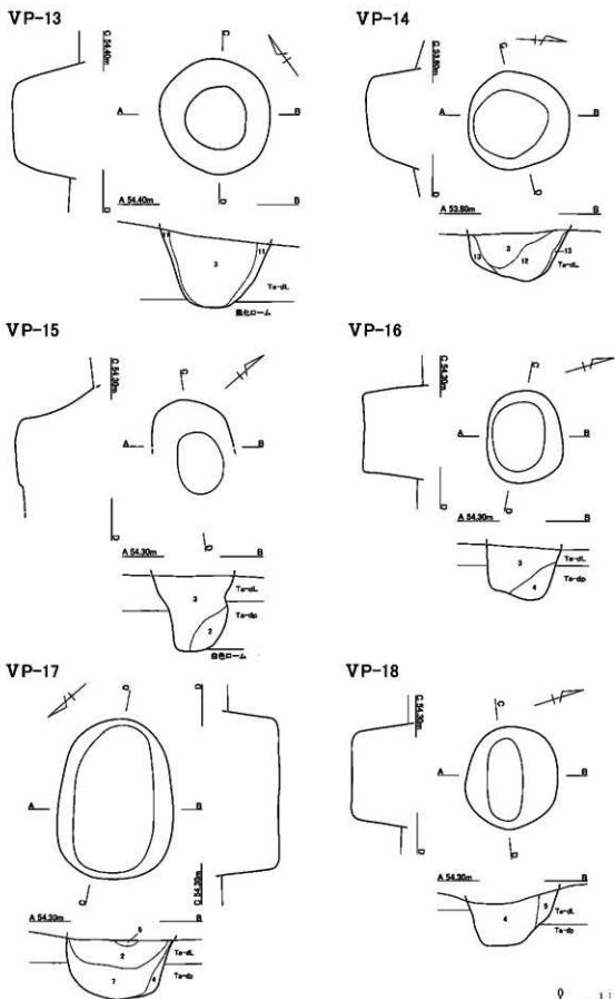
図Ⅲ-2 VP-13～18 平面及び断面図
