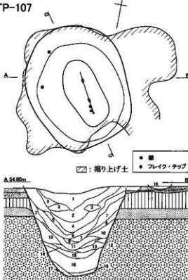
図Ⅲ-9 TP-106・107 平面及び断面図
