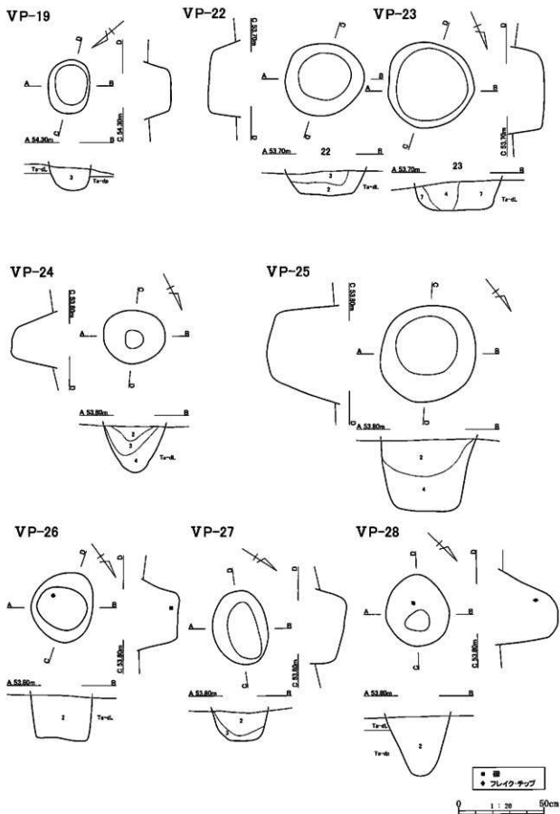
図Ⅲ-3 VP-19・22～28 平面及び断面図
