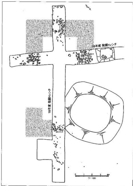
第6図 中堂救世殿面の平面図 (1:133)
