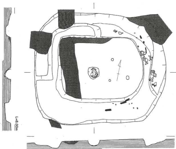
第14图 東五反田遺跡方形周溝墓実測図(1/80)
