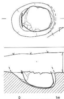
第17図 東若宮遺跡出土土壺棺墓実測図(1/30)
