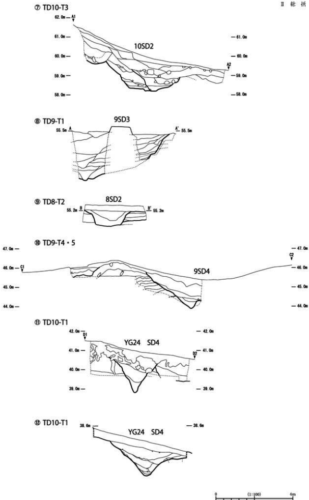
図11 堰跡の断面図（II期）・その他
