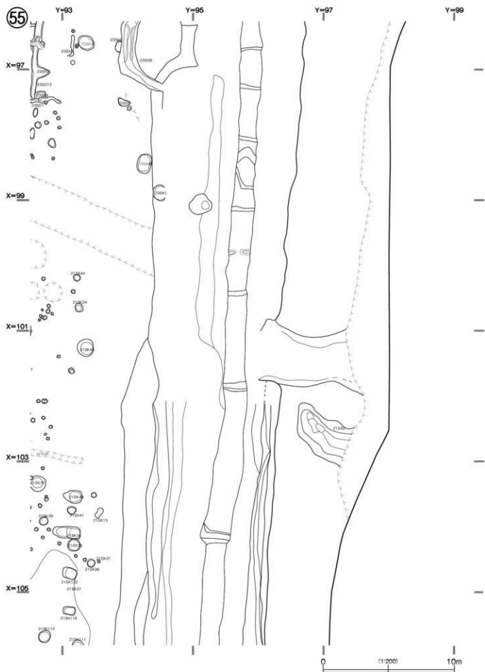
图63 遺構平面図55 (1/200)
