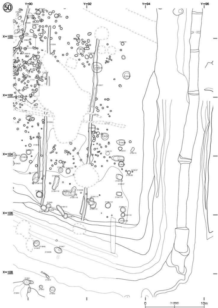
図58 遺構平面図50 (1/200)
