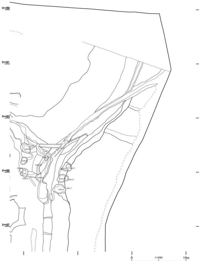
図62 遺構平面図54 (1/200)
