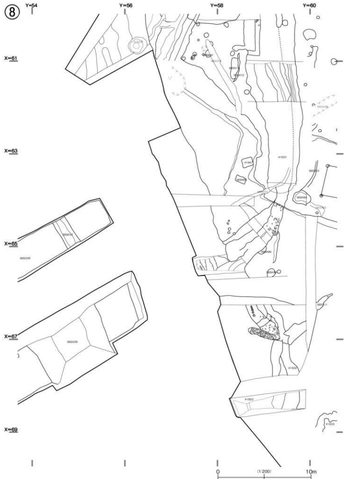
図16 遺構平面図⑧ (1/200)
