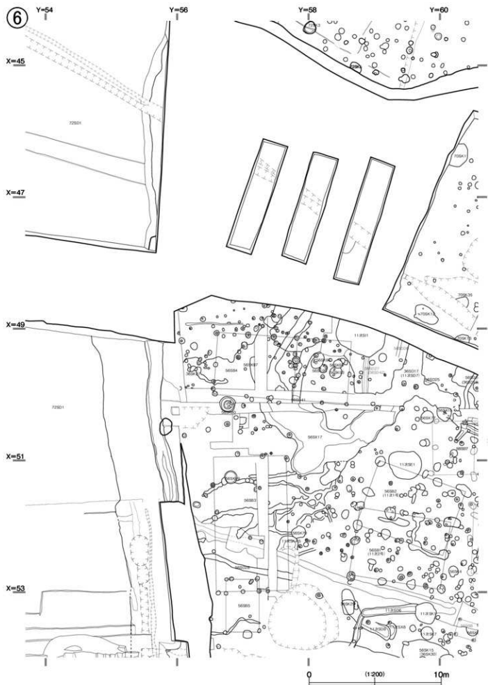
図14 遺構平面図⑥ (1/200)
