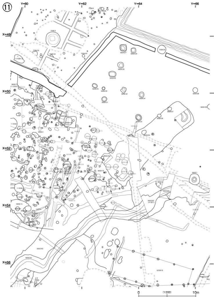
図19 遺構平面図⑪ (1/200)
