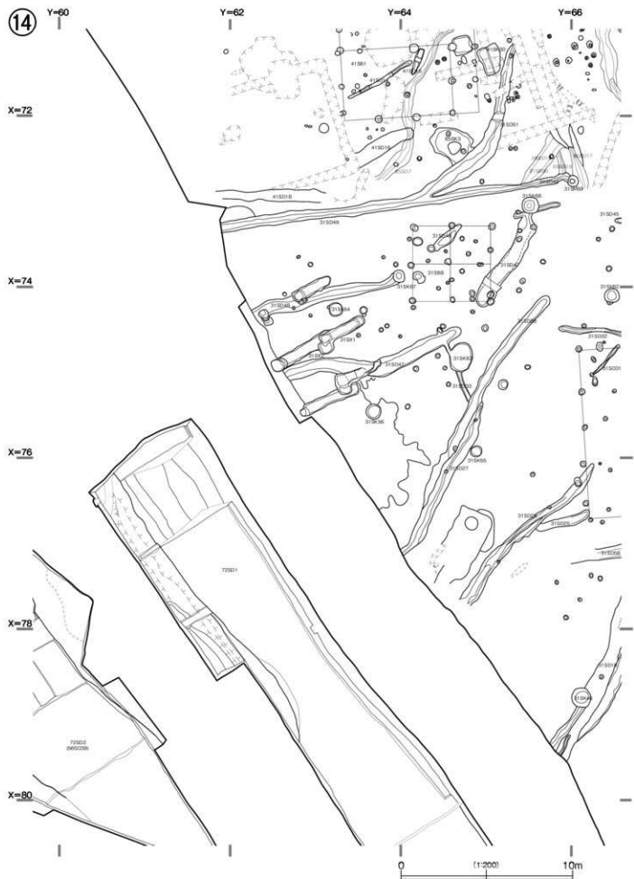
図22 遺構平面図⑭ (1/200)
