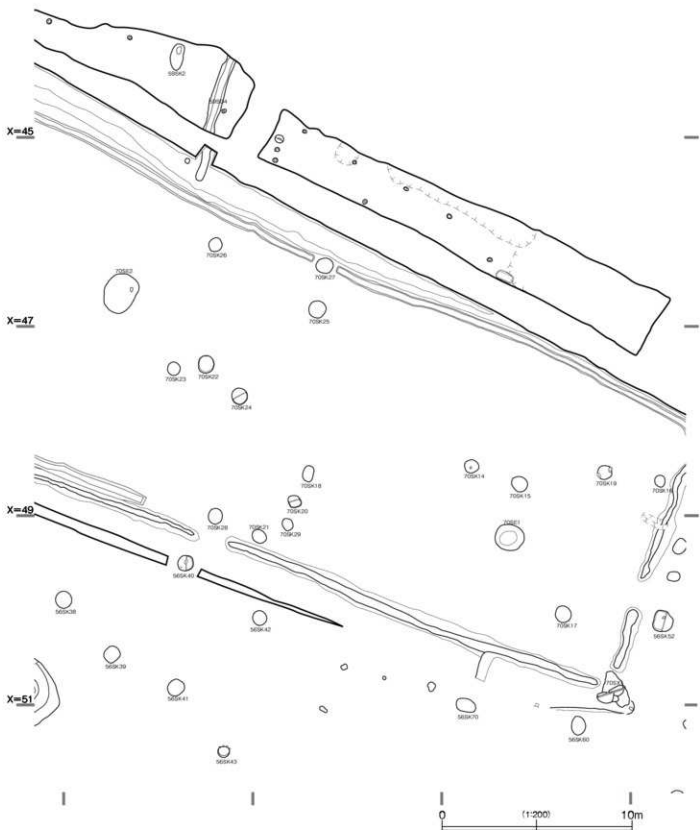
図24 遺構平面図⑬ (1/200)
