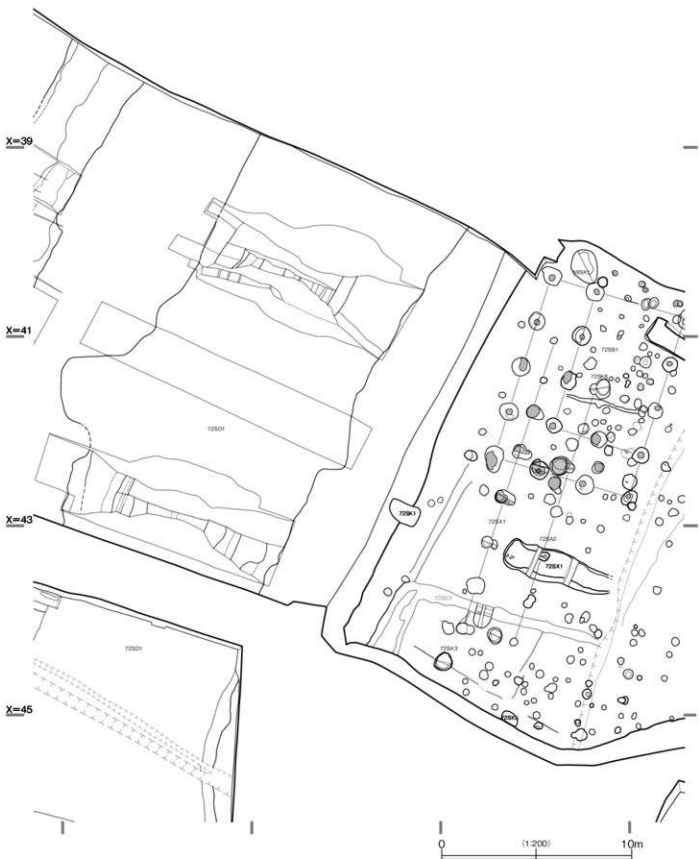
図13 遺構平面図⑤ (1/200)
