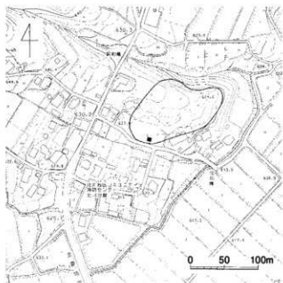
図35 北屋敷遺跡 範囲と調査地
