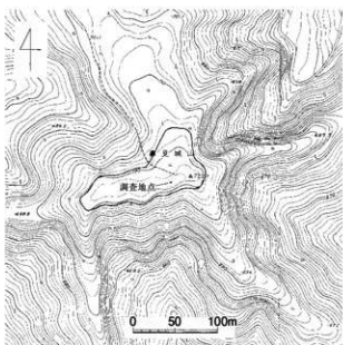
図33 鼻見城跡 範囲と調査地
