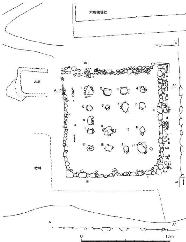
第 15 圖 講堂跡実測圖 (1 / 200)
