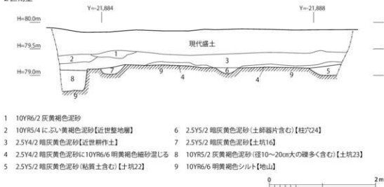
図10 2区壁面断面図(1:50)
