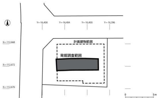
図4 調査区配置図 (1:200)
