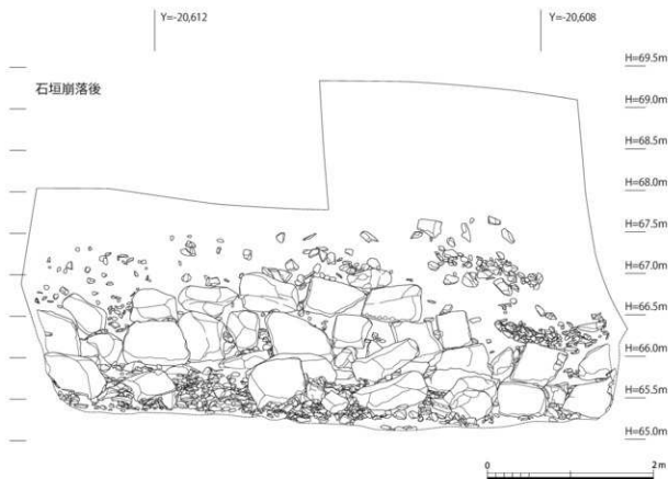
図16 4区立面図 (1 : 50)
