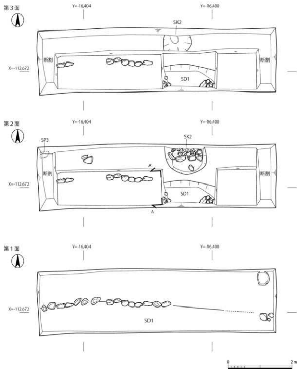
图7 各遺構面平面図 (1:60)
