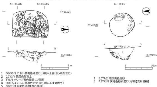
図8 土坑2 平・断面図 (1:40)
