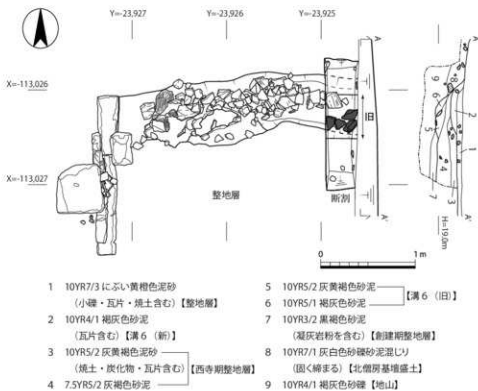
図12 溝6 (新・旧) 実測図 (1 : 40)
