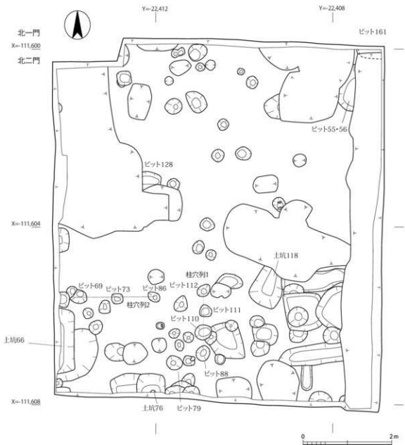
図8 第2面平面図 (1:60)
