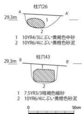
図13 柱穴26、43断面図 (1:20)
