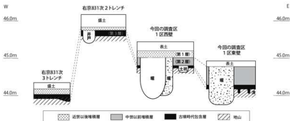
図6 基本層序模式図
