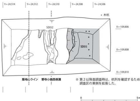
図9 北区遺構平面図(1:100)
