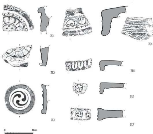
図21 出土瓦実測図及び拓影(1:4)
