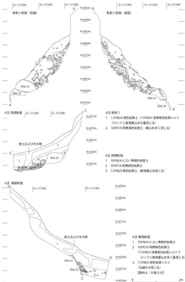
図17 4区調査区壁及び断削2断面図 (1:50)
