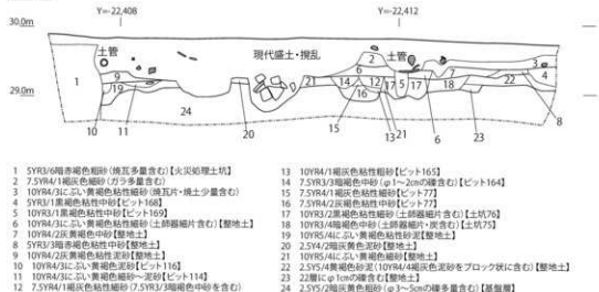
図5 調査区断面図 (1:60)
