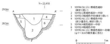
図7 井戸152断面図 (1:40)
