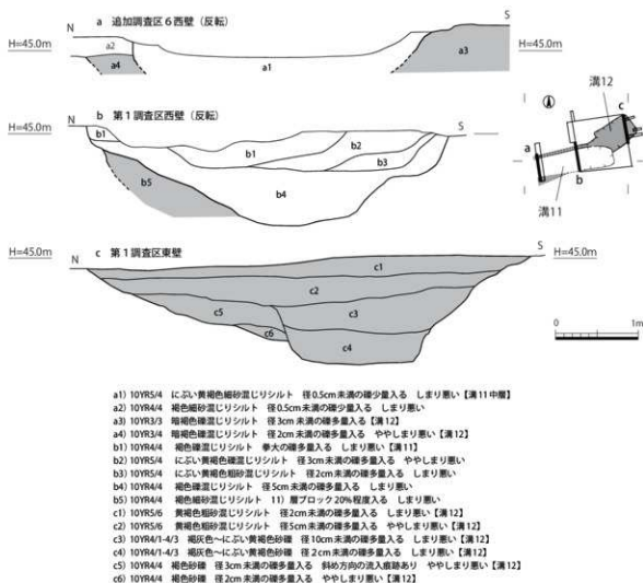
図12 溝11断面図（1：50）
