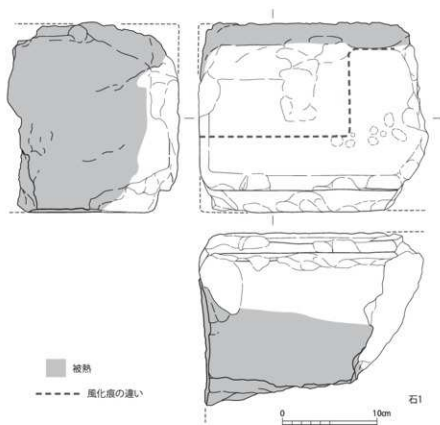
図16 石製品実測図（1：4）
