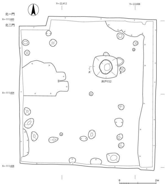
図6 第3面平面図 (1:60)
