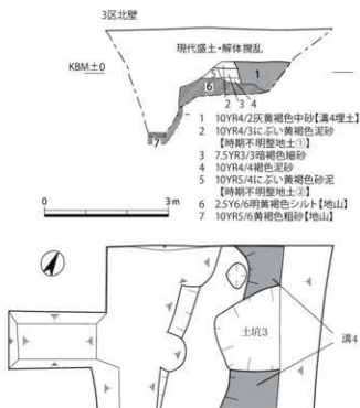
図36 3区平・断面図 (1:100)
