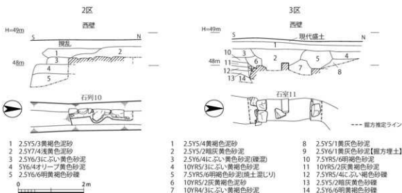
図6 2・3区平・断面図 (1:80)
