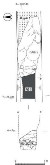
図5 石垣平・立面図 (1:40)
