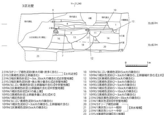
図41 3区断面図 (1:50)
