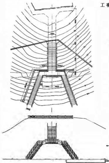
工事平面図
