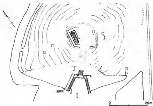
工事平面図
