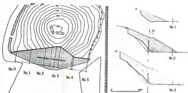
図79 稲荷山古墳 昭和57年度工事の平面及び造成法面横断面
