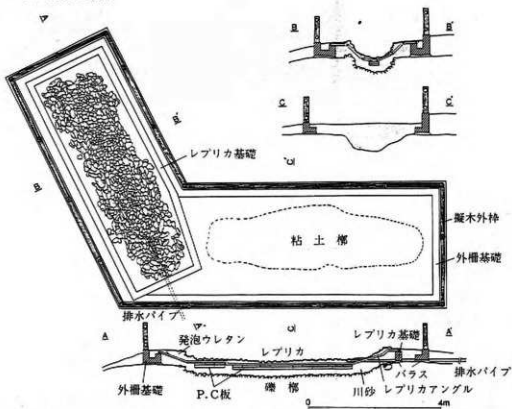
図80 稲荷山古墳 昭和58年度工事における主体部防護柵及び礫層レプリカの設置
