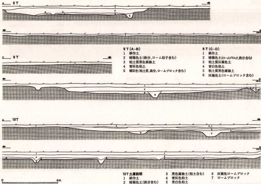
第11図 昭和42年度第9、第10トレンチ(A-B)土層断面図(1/80)
