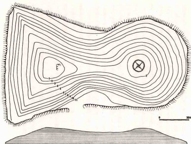
第1図 二子山古墳測量図（1/800 昭和12年 後藤守一、三木文雄氏原図、「古墳調査報告書 第六編」埼玉県教育委員会 昭和39年、より転載）
