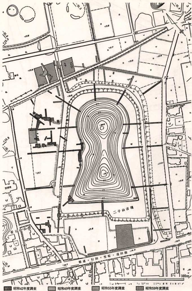
第3圖 二子山古墳各年度毎発掘調査位置 (1/1,500)
