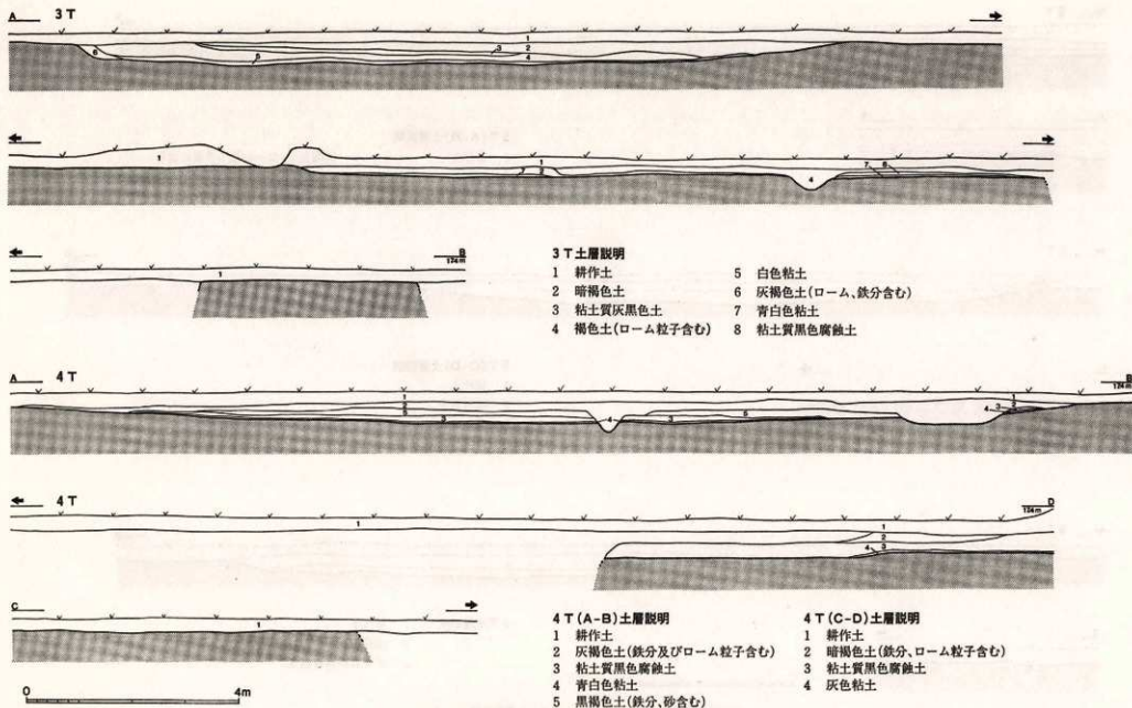
第9図 昭和42年度第3、第4トレンチ土層断面図(1/80)
