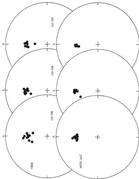
第41図 各サイトごとの各試料の消磁前と交差消磁後の残留化方向の等面積投影図
