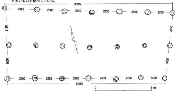
図5 中門～5溝付近検出建物
