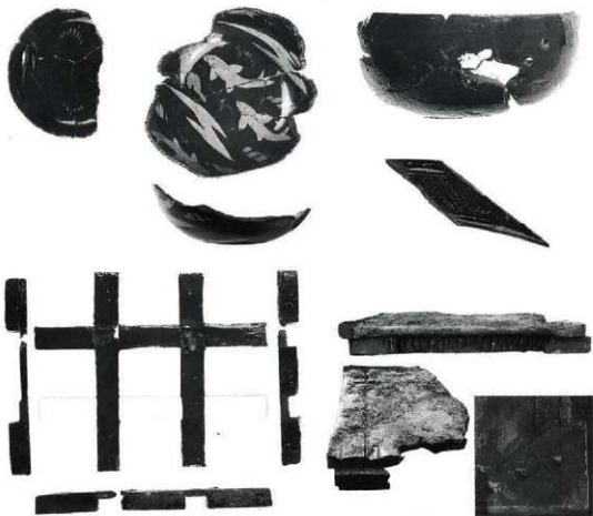
井桁状組物（組み方は推定）
