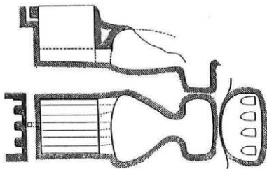
水殿瓦窯跡 (『埼玉県史』より転載) S=1/50
