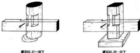
図4 掘立柱・横木組合模式図
