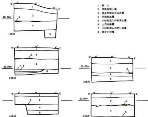
図6 北部地区試掘土層図
