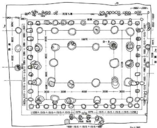
図5 薬師堂及び廊配置模式図
