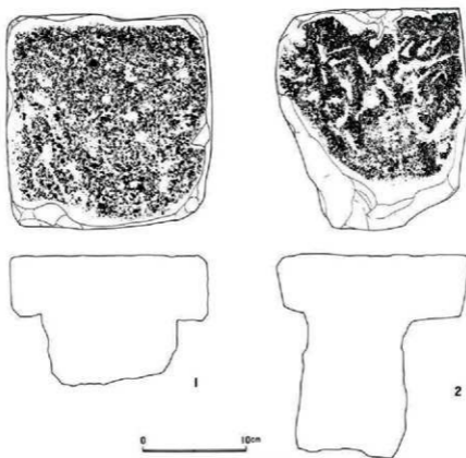
図21 壇上積基壇東石
