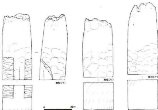
図3 木造基壇束柱
