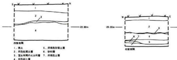
図2 61年度調査区標準土層柱状図
