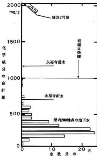
図18 化学成分の合計量の度数分布——栗内200地点の地下水および永福寺湧水、周辺の地下水等 永福寺湧水、鎌倉2号泉、永福寺沢水は、栗内の地下水と比較して化学成分の合計量が多いことが判る。
