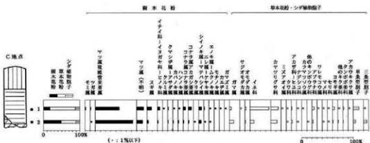
図22 C地点の主要花粉化石分布図
