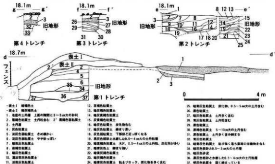
図6 トレンチセクション図
