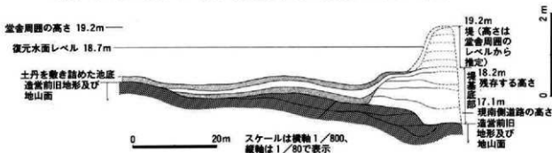
図17 池底断面模式図
