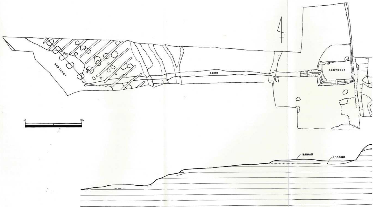
第9圖 T8705調査地実測図 (1/200)
