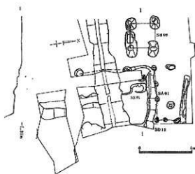
SBOB・SA01実測図 (1/200)
