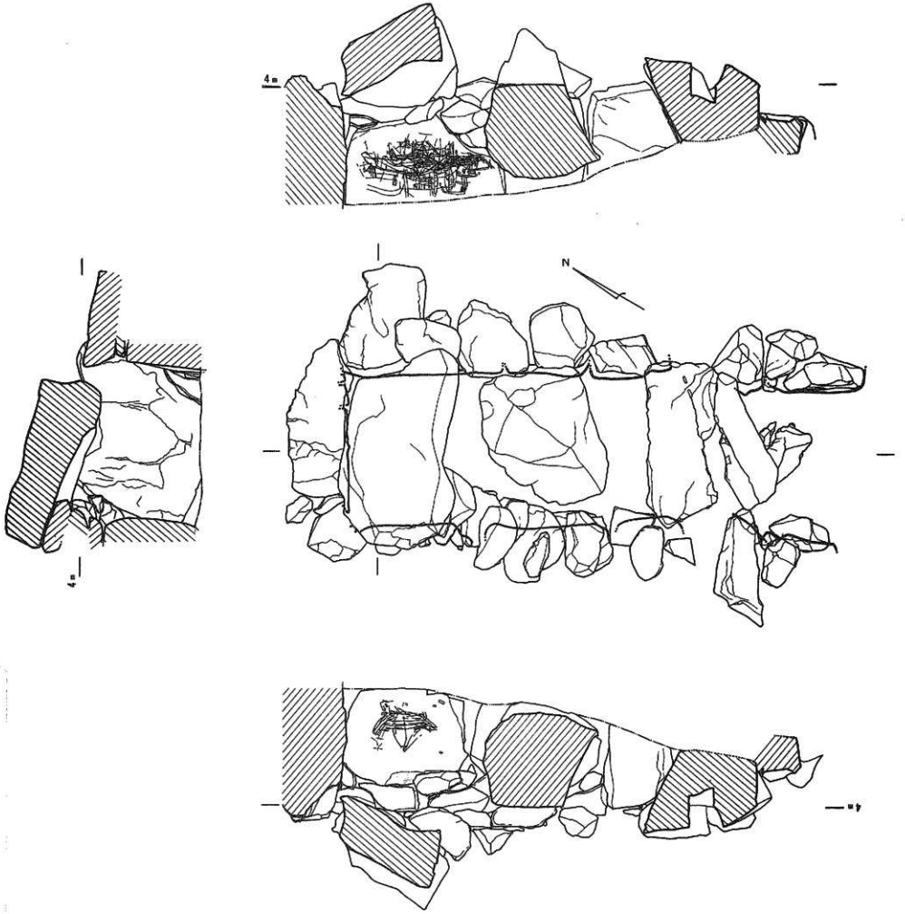
Fig5 石室実測図 (縮尺1/40)
