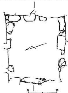
第5図 玄室根石配置図
