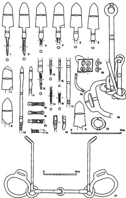
第10图 玄室出土遺物実測图(2)
