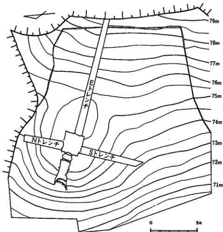
第3図 墳丘測量図
