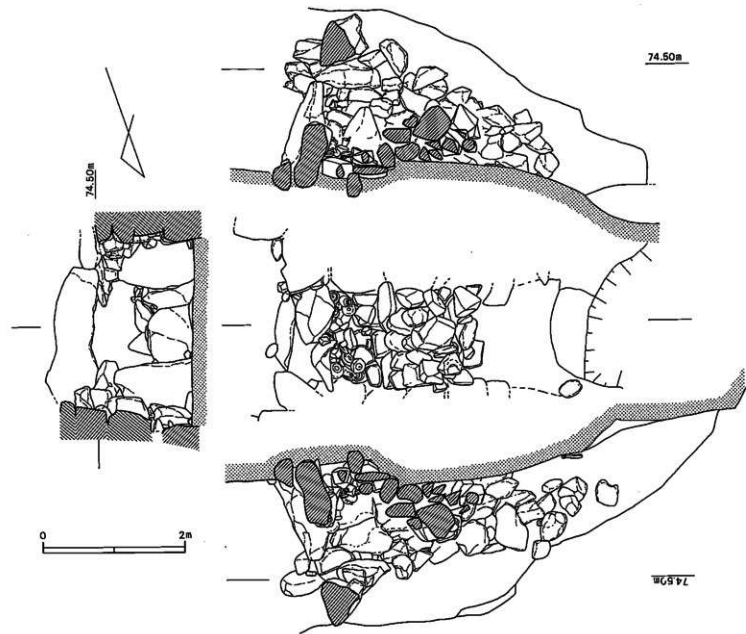
第7圖 渡道閉塞狀況圖
