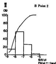
図21 レキの粒径分布 (2) ヒストグラムおよび粒径加積曲線
