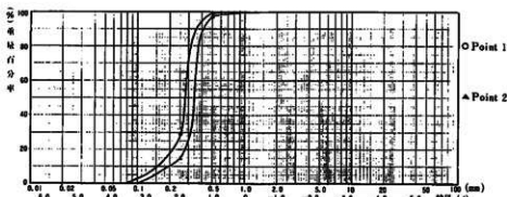
図22 matrix 部の粒度分布 (1) 粒径加積曲線 \Phi(\phi) = -\log \phi
