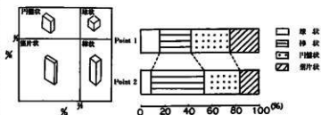
図25 レキの形状分類とその個数比
