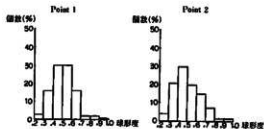
図27 レキの球形度分布 (1) ヒストグラム
