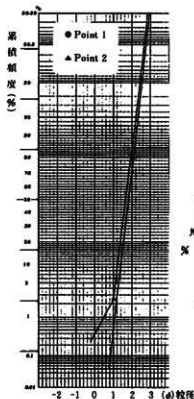
図23 matrix 部の鉱物組成 (2) 標準累級曲線 (正規標準率による)
