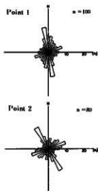
図29 レキの長軸の配列方向のローズダイヤグラム
