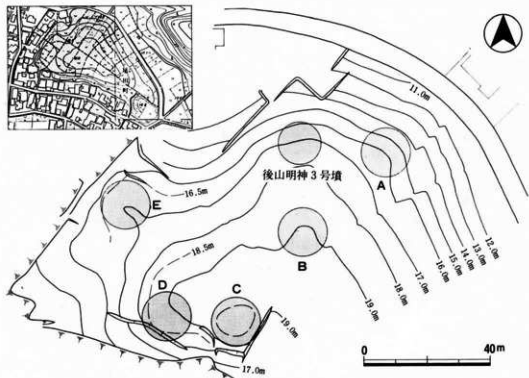
第6図 埴田後山古墳群測量図（S-1/1200）
