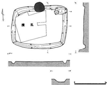
第9图 68A号住居跡 (1/60)
