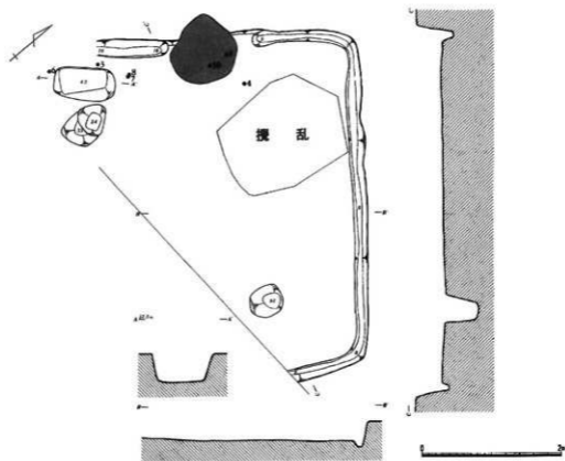
第16図 71号住居跡 (1/60)
