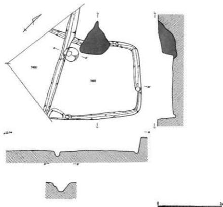
第15図 70・74号住居跡 (1/60)
