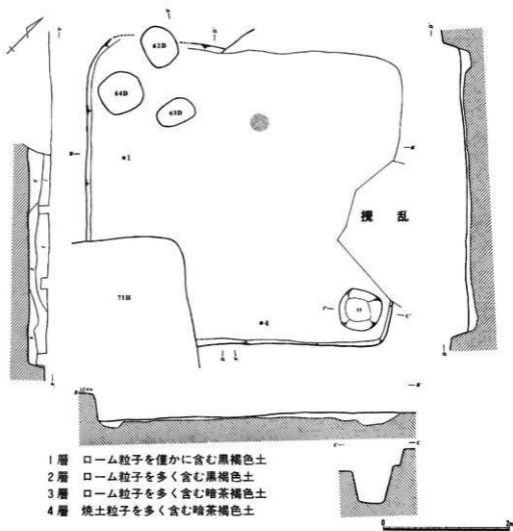
第19図 72号住居跡 (1/60)
