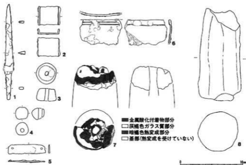
第26図 住居跡出土土製品・鉄製品 (1/3)
