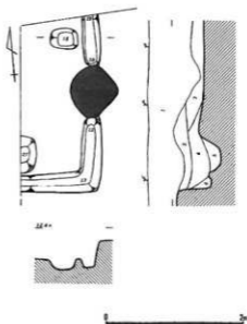
第24図 75号住居跡 (1/60)
