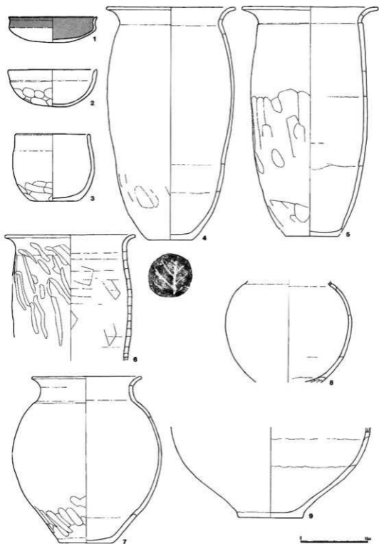
第17图 71号住居跡出土遺物1 (1/4)
