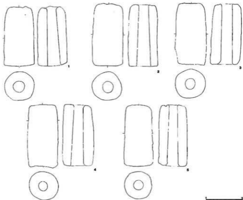
第28図 63号土坑出土遺物 (1/5)
