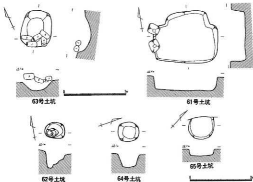
第27図 土坑 (61・62・64・65号土坑=1/60, 63号土坑=1/30)
