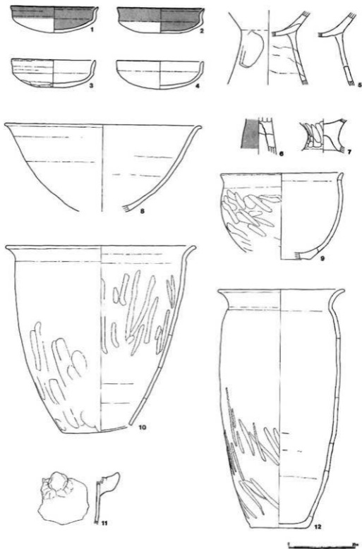
第22図 73号住居跡出土遺物1 (1/4)
