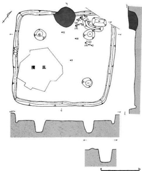
第12図 69号住居跡 (1/60)
