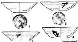
第16図 52号土坑出土遺物 (1/4)
