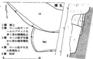
第6図 1号住居跡、50号土坑（1/60）
