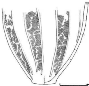
第5図 1号埋壘埋設土器 (1/4)
