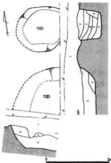
第14図 51・52号土坑(1/60)
