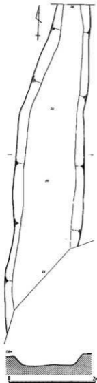
第20図 2号溝跡 (1/60)
