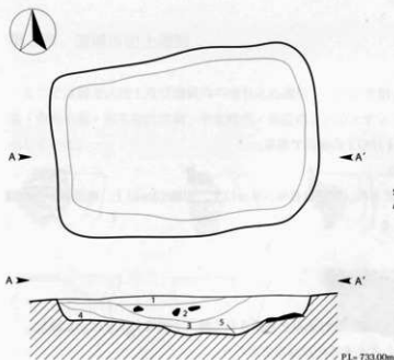
第10図 SK01実測図 (1/30)
