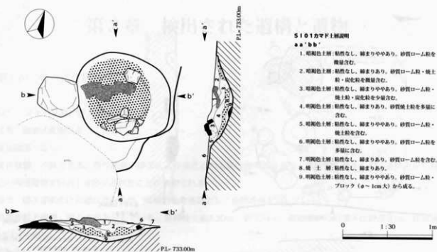
第6図 SI01カマド実測図 (1/30)
