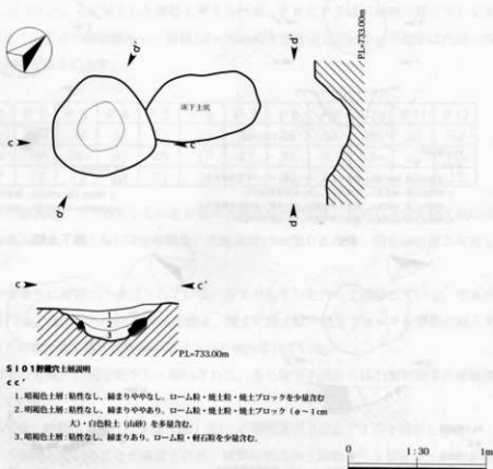
第7図 SI01貯蔵穴実測図 (1/30)
