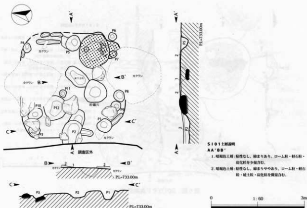
第4図 SI01実測図 (1/60)
