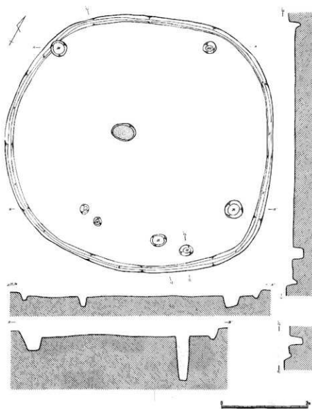
第54図 254号住居跡(1/60)
