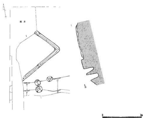
第4图 7号住居跡 (1/60)
