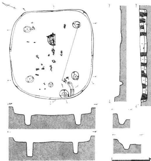
第49図 252号住居跡 (1/60)
