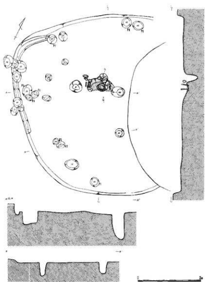
第8图 28号住居跡 (1/60)
