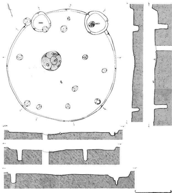
第12図 65号住居跡(1/60)
