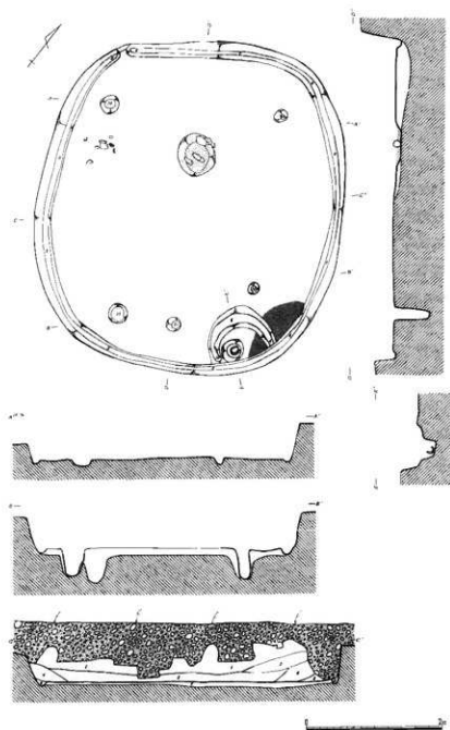
第44図 131号住居跡 (1/60)
