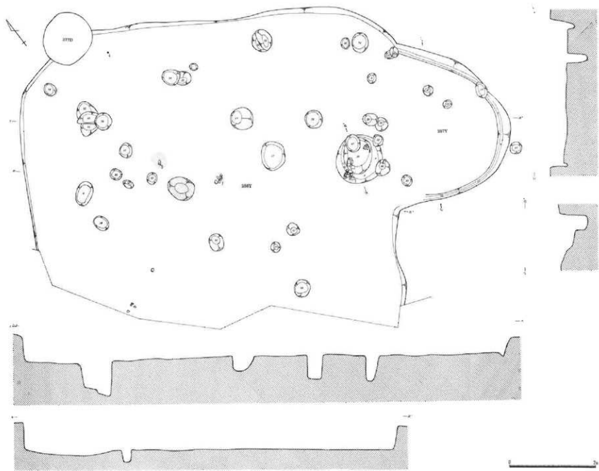
第55图 255・257号住居跡 (1/60)
