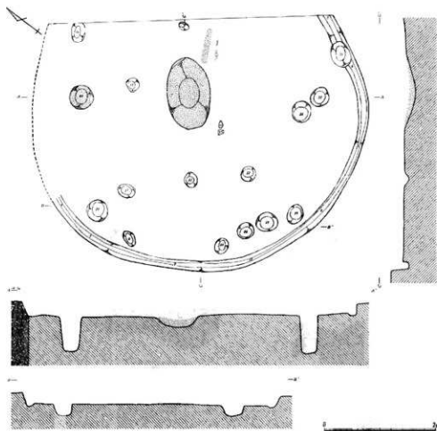
第52図 253号住居跡(1/60)
