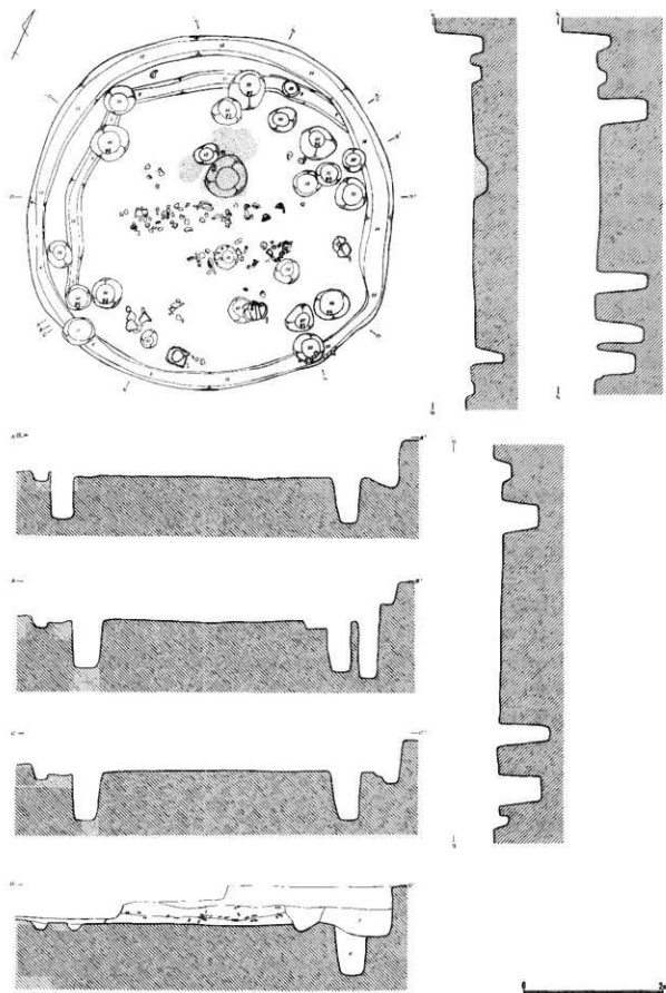
第31图 74号住居跡 (1/60)
