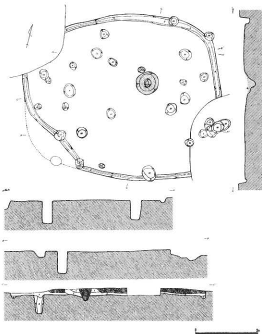
第29図 73号住居跡 (1/60)
