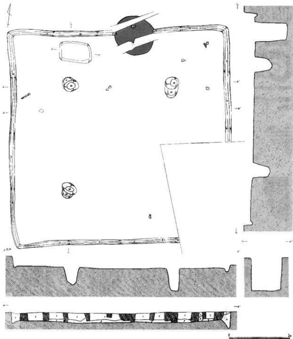
第65図 13号住居跡(1/60)
