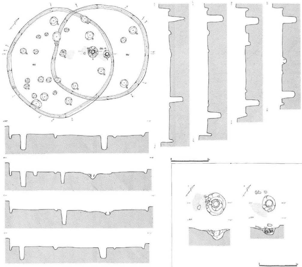
第18图 68·70号住居跡 (1/60)、炉跡 (1/30)
