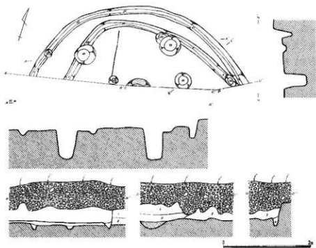
第15図 66号住居跡 (1/60)
