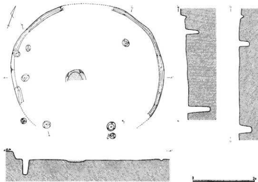
第58図 256号住居跡（1/60）
