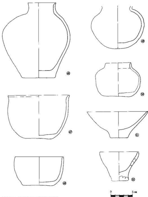
第8図 團横穴墓出土遺物実測図
