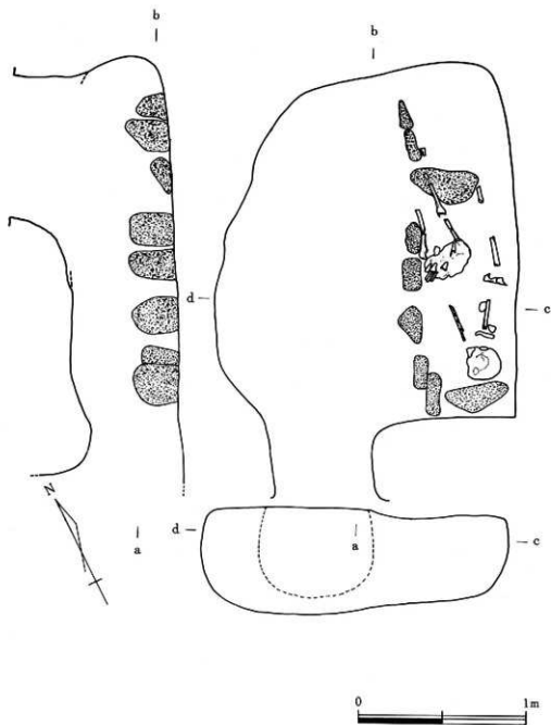
第3图 元地原地下式第2号墳実測图
