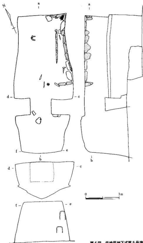
第6图 元地原地下式第5号填塞测图
