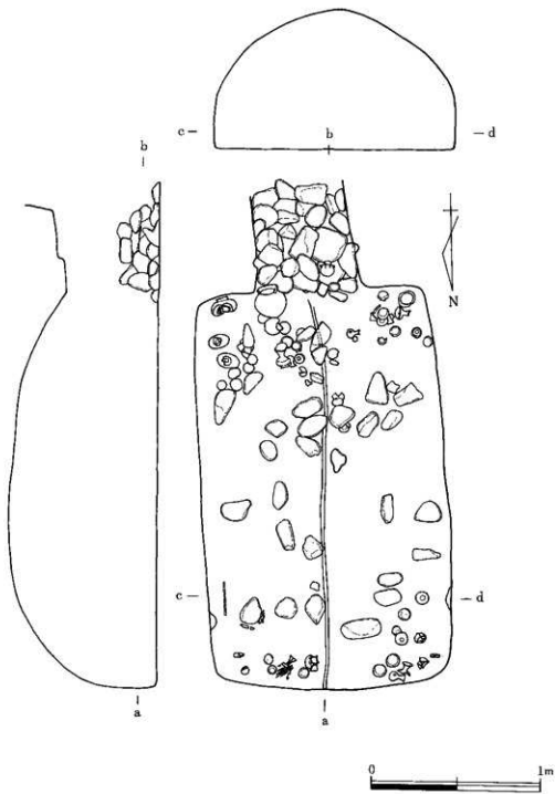
第1图 圆横穴墓实测图
