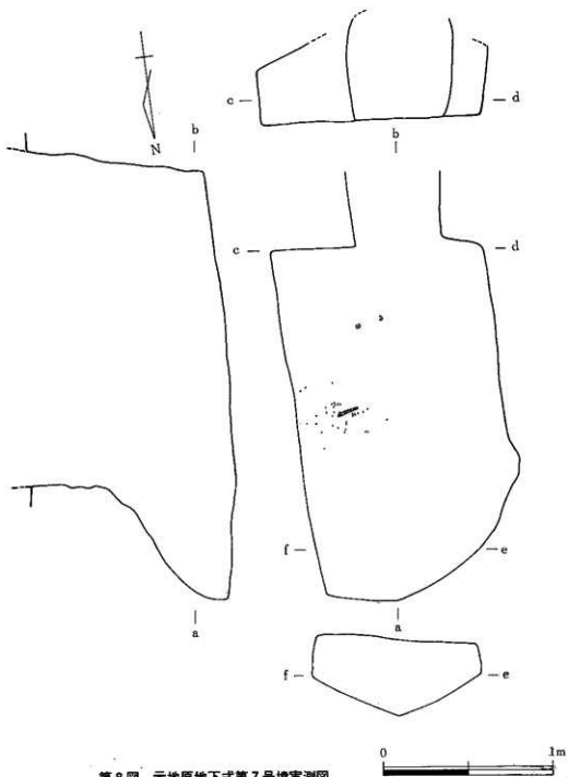
第 8 图 元地原地下式第 7 号填实测图
